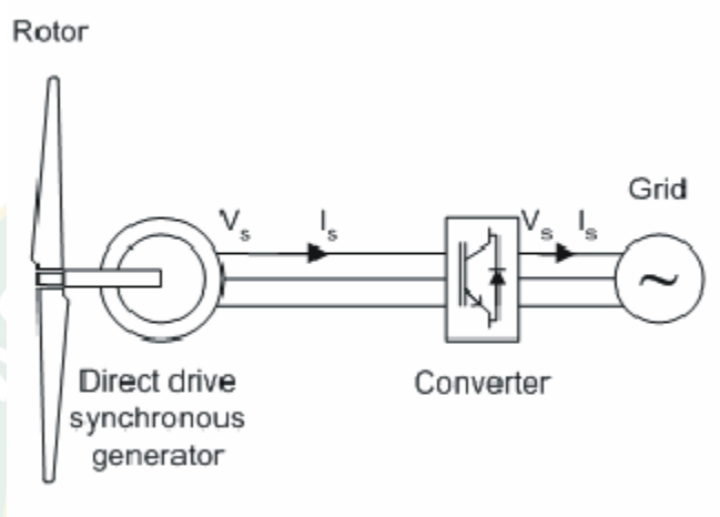
ภาพที่ 14 แสดง Variable speed based on a direct drive and synchronous generator
