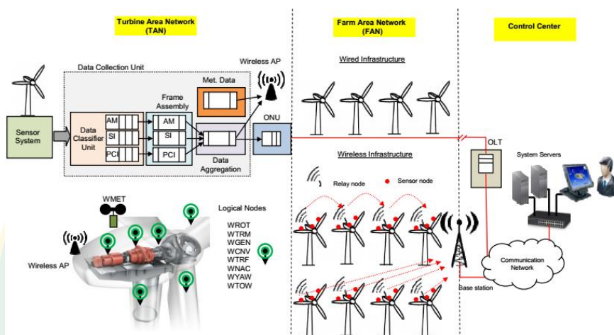
ภาพที่ 21 การสื่อสารแบบ M2M
