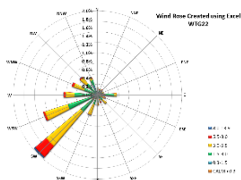
ภาพที่ 28 ลักษณะลมพัดผ่านกังหันลมหมายเลขที่ WTG 22 เดือนมีนาคม-กันยายน
