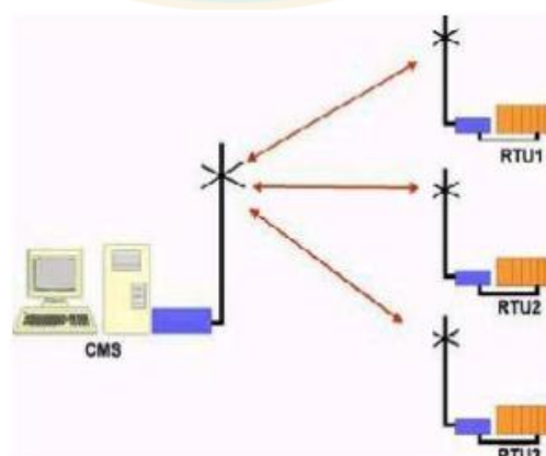
ภาพที่ 19 Point-to-Multipoint Configuration
