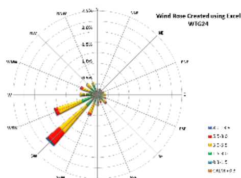
ภาพที่ 32 ลักษณะลมพัดผ่านกังหันลมหมายเลขที่ WTG 24 เดือนมีนาคม-กันยายน
