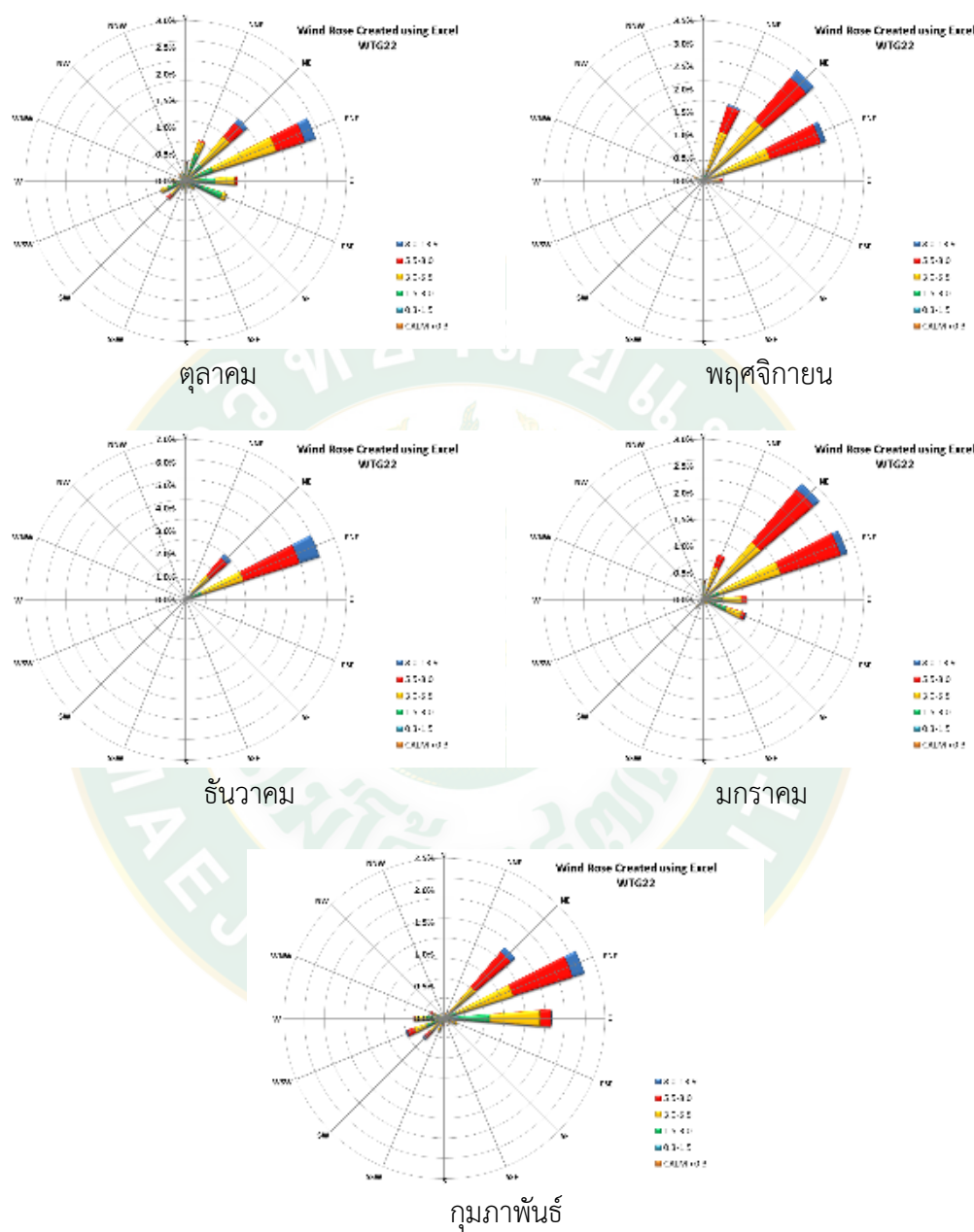
ภาพที่ 29 ลักษณะลมพัดผ่านกังหันลมหมายเลขที่ WTG 22 เดือนตุลาคม-กุมภาพันธ์
