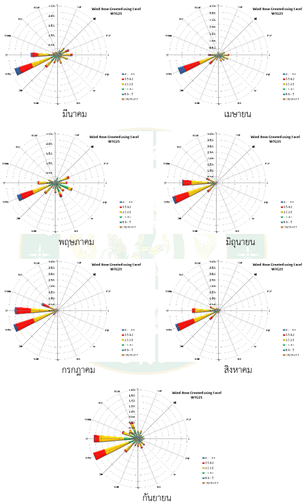
ภาพที่ 26 ลักษณะลมพัดผ่านกังหันลมหมายเลขที่ WTG 21 เดือนมกราคม-กันยายน
