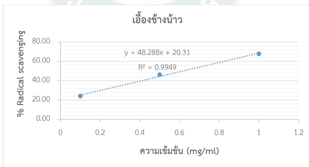
ภาพภาคผนวกที่ 3 กราฟ %Radical scavenging ของ เอื้องช้างน้าว ด้วยวิธี ABTS
