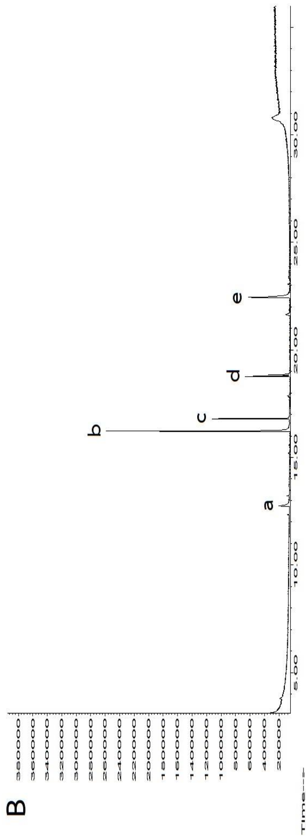
ภาพที่ 28 GC-MS spectra ของสารสกัดหยาบจากลำต้นเอื้องมัจฉาเหลือทิ้งที่ทำการสกัดด้วย 60% เอทานอล
