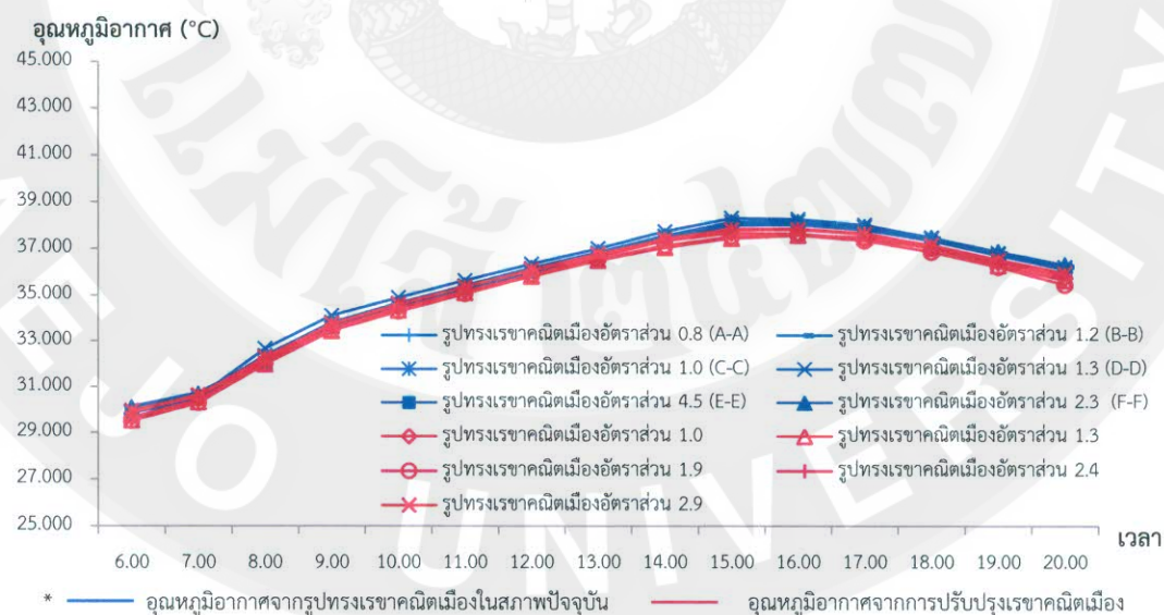
ภาพที่ 148 แสดงการเปรียบเทียบการเปลี่ยนแปลงอุณหภูมิอากาศ ในช่วงเวลา 6.00 – 20.00 น. ระหว่างรูปทรงเรขาคณิตเมืองในสภาพปัจจุบัน และปรับปรุงรูปทรงเรขาคณิตเมือง ในแนวนอนทิศเหนือ – ทิศใต้
