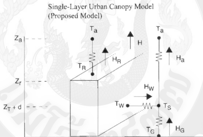
ภาพที่ 52 รูปแบบการคำนวณฟลักซ์และอุณหภูมิของพลังงานสำหรับแบบจำลอง SLUCM ที่มา : Kusaka et al. (2001)
