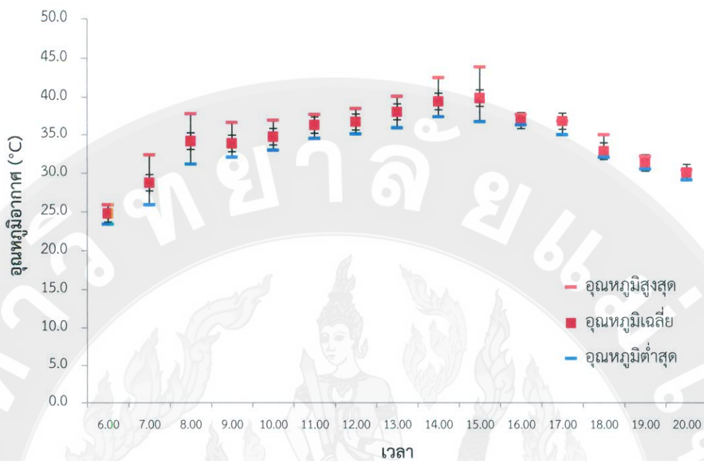
ภาพที่ 81 แผนภูมิแสดงอุณหภูมิอากาศ วันที่ 24 - 25 เมษายน 2560 ณ จุดตรวจวัดสภาพอากาศ วัดศรีดอนไชย
