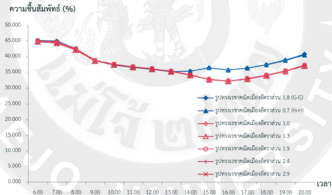
ภาพที่ 151 แสดงการเปรียบเทียบการเปลี่ยนแปลงความชื้นสัมพัทธ์ ในช่วงเวลา 6.00 – 20.00 น. ระหว่างรูปทรงเรขาคณิตเมืองในสภาพปัจจุบัน และปรับปรุงรูปทรงเรขาคณิตเมือง ในแนวนอนทิศตะวันออก – ทิศตะวันตก
