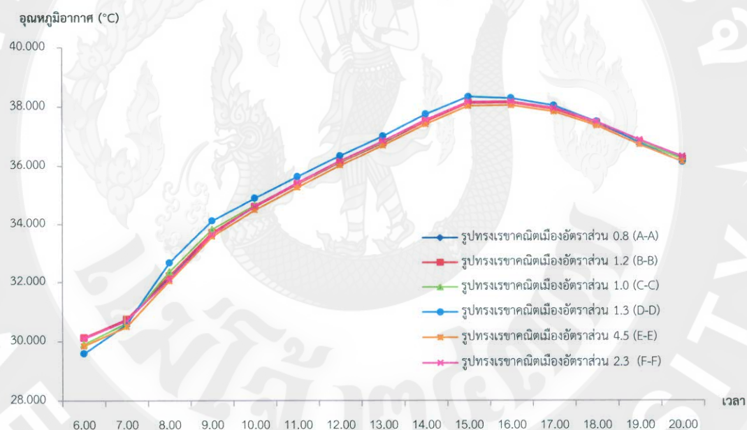
ภาพที่ 123 แสดงแผนภูมิอุณหภูมิอากาศปัจจุบัน บริเวณจุดตัวอย่างรูปทรงเรขาคณิตเมือง ตามแนวถนนเหนือ - ใต้
