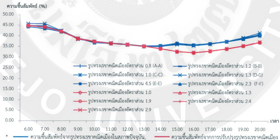
ภาพที่ 150 แสดงการเปรียบเทียบการเปลี่ยนแปลงความชื้นสัมพัทธ์ ในช่วงเวลา 6.00 – 20.00 น. ระหว่างรูปทรงเรขาคณิตเมืองในสภาพปัจจุบัน และปรับปรุงรูปทรงเรขาคณิตเมือง ในแนวนอนทิศเหนือ – ทิศใต้
