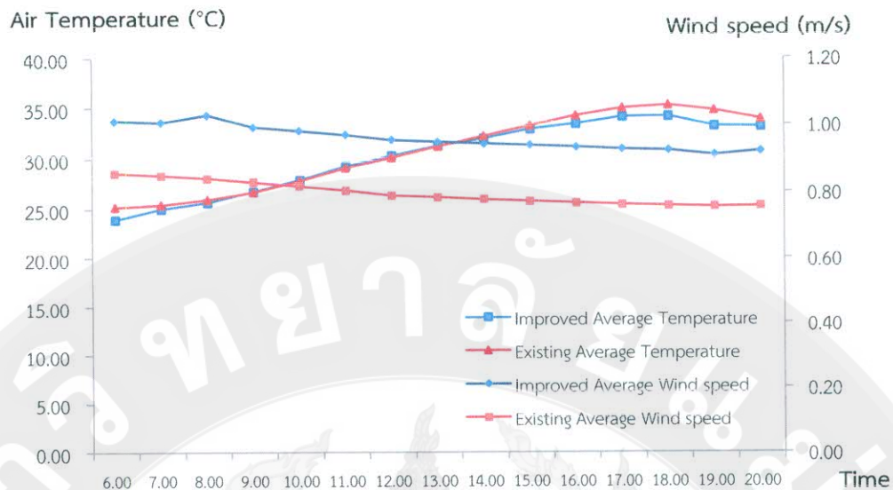
ภาพที่ 12 แสดงแผนภูมิการเปรียบเทียบการเปลี่ยนแปลงของอุณหภูมิและความเร็วลม ในพื้นที่ศึกษาสภาพปัจจุบัน และในกรณีการเปิดช่องระบายอากาศบางส่วนในพื้นที่ชั้นหนึ่งของอาคาร
