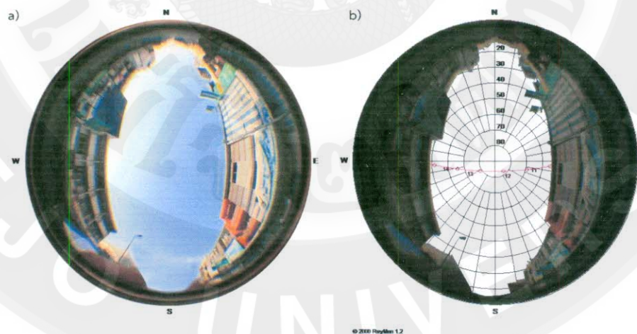
ภาพที่ 109 a) Sky view factor บริเวณกลางถนนของรูปทรงเรขาคณิตเมืองอัตราส่วน 0.40 b) ช่วงเวลาได้รับแสงอาทิตย์ของจุดรูปทรงเรขาคณิตเมืองอัตราส่วน 1.2 ที่มา : ผู้วิจัย
