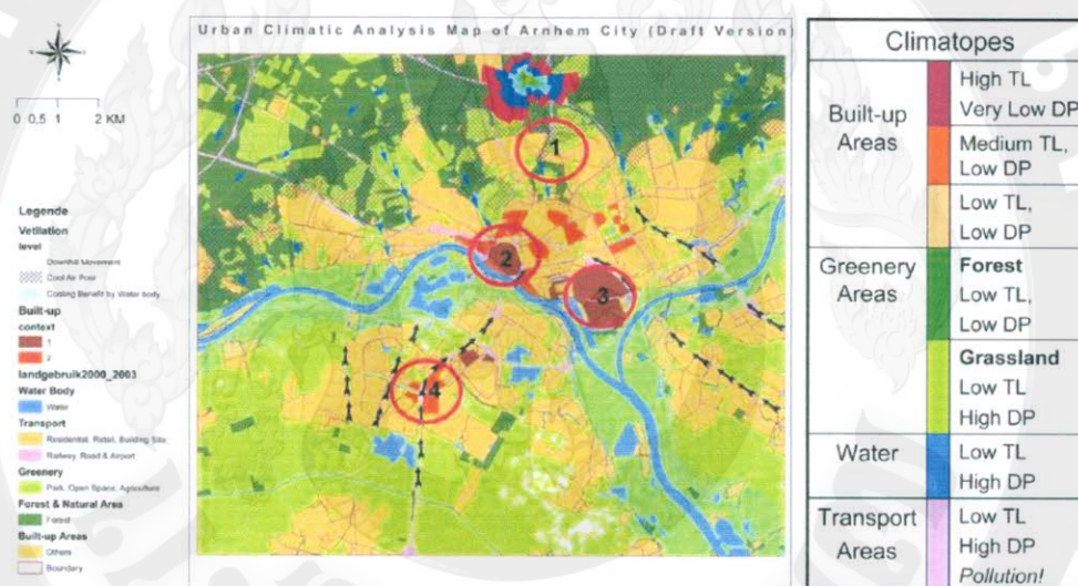
ภาพที่ 12 แสดงภาพ UC-AnMap for Arnhem with the legend of climatopes and four designated areas (TL means thermal load; DP means dynamic potential).
