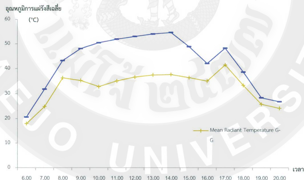
ภาพที่ 138 แสดงอุณหภูมิการแผ่รังสีปัจจุบัน บริเวณจุดตัวอย่างรูปทรงเรขาคณิตเมือง ตาม แนวถนนตะวันออก – ตะวันตก
