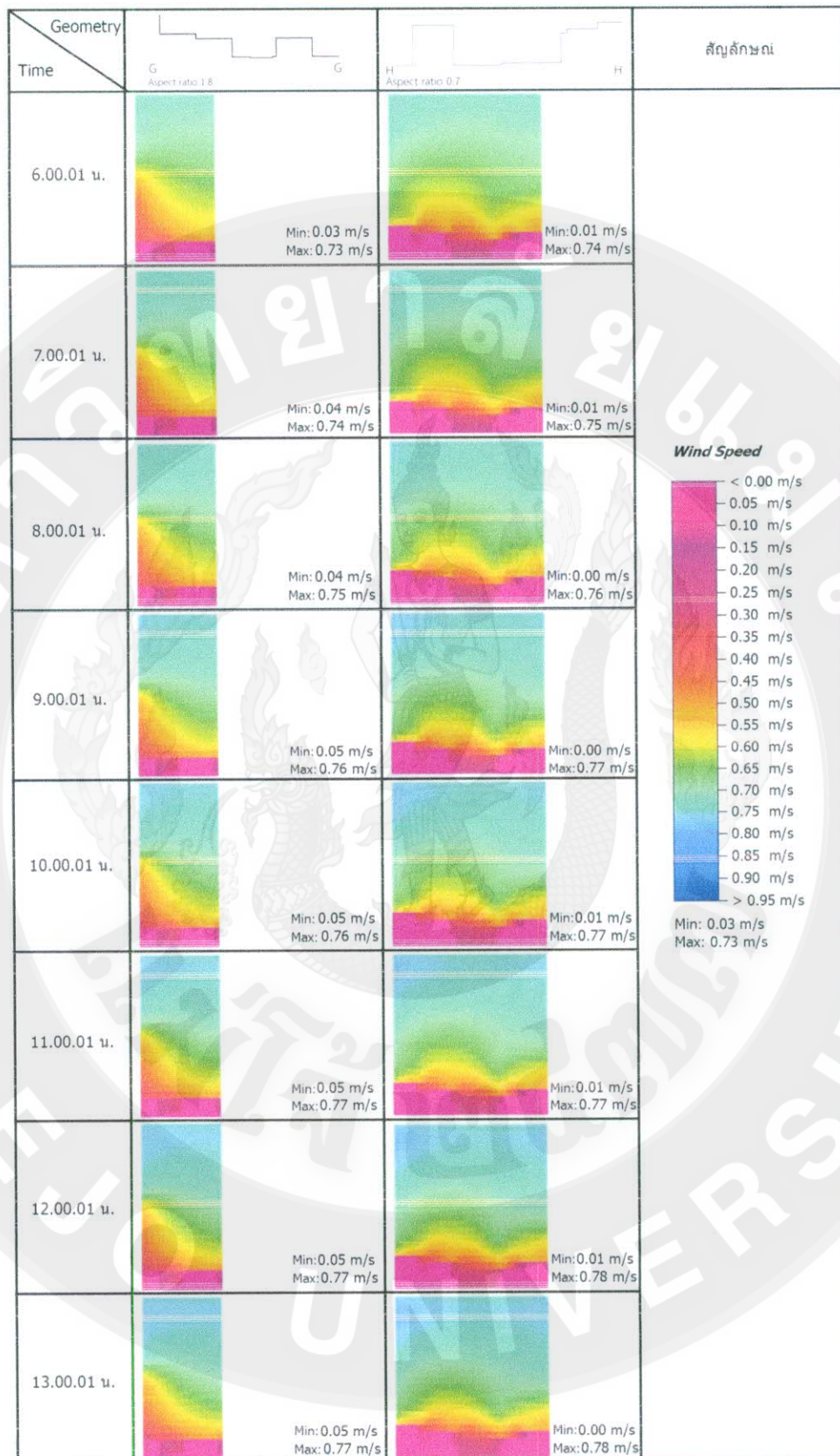
ภาพแสดงความเร็วลม(m/s) ของรูปทรงเรขาคณิตเมือง 1.8 และ 0.7 ในสภาพปัจจุบัน บริเวณถนนเหนือพื้นดิน 1.80 เมตร ตามถนนทิศตะวันออก-ทิศตะวันตก เวลา 6.00-13.00 น.
