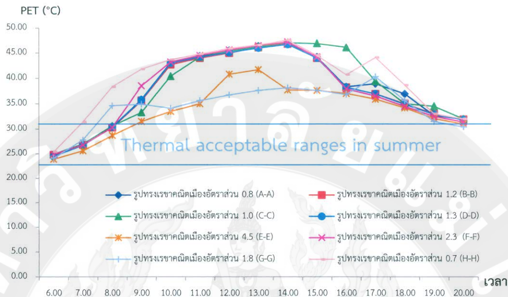
ภาพที่ 140 แสดงอุณหภูมิสมมูลทางสรีรวิทยาจากอิทธิพลรูปทรงเรขาคณิตเมืองในสภาพปัจจุบัน ที่มา : ผู้วิจัย
