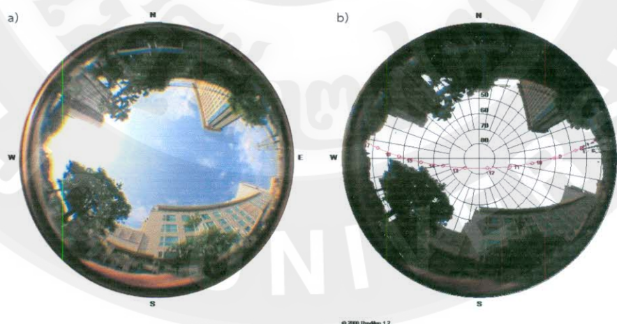
ภาพที่ 122 a) Sky view factor บริเวณกลางถนนของรูปทรงเรขาคณิตเมืองอัตราส่วน 0.35 b) ช่วงเวลาได้รับแสงอาทิตย์ของจุดรูปทรงเรขาคณิตเมืองอัตราส่วน 0.7
