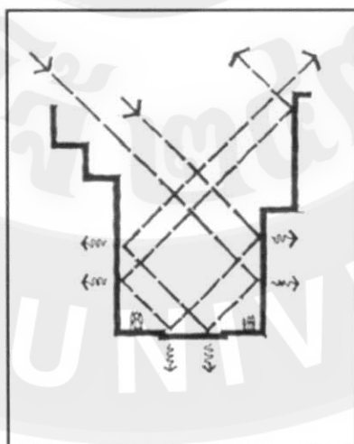
ภาพที่ 17 แสดงการสะท้อนและกักเก็บความร้อนจากการแผ่รังสีของดวงอาทิตย์ในพื้นที่ถนนระหว่างอาคาร (Street canyon หรือ Urban canyon) ในเวลากลางวัน
