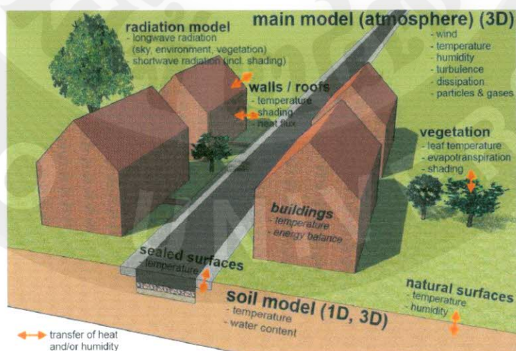
ภาพที่ 45 แสดงตัวแปร และสมการย่อยของโปรแกรม ENVI-Met
