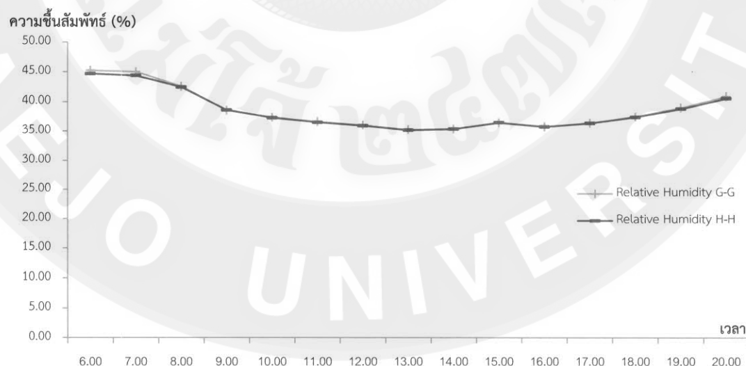
ภาพที่ 127 แสดงความชื้นสัมพัทธ์ปัจจุบัน บริเวณจุดตัวอย่างรูปทรงเรขาคณิตเมือง ตามแนวถนนตะวันออก – ตะวันตก
