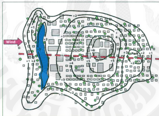
ภาพที่ 29 แผนที่เส้นชั้นอุณหภูมิเท่า แสดงให้เห็นถึงปรากฏการณ์ UHI ในบรรยากาศในช่วงกลางคืน ที่มา : Wong (2008)
