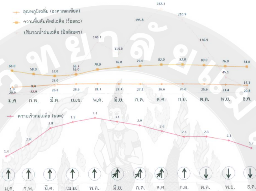
ภาพที่ 5 แสดงลักษณะภูมิอากาศจากสถิติภูมิอากาศในคาบ 30 ปี ของจังหวัดเชียงใหม่
