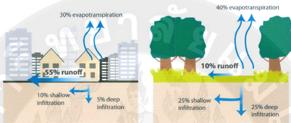
ภาพที่ 24 แสดงลักษณะพื้นผิว และกระบวนการคายระเหย
