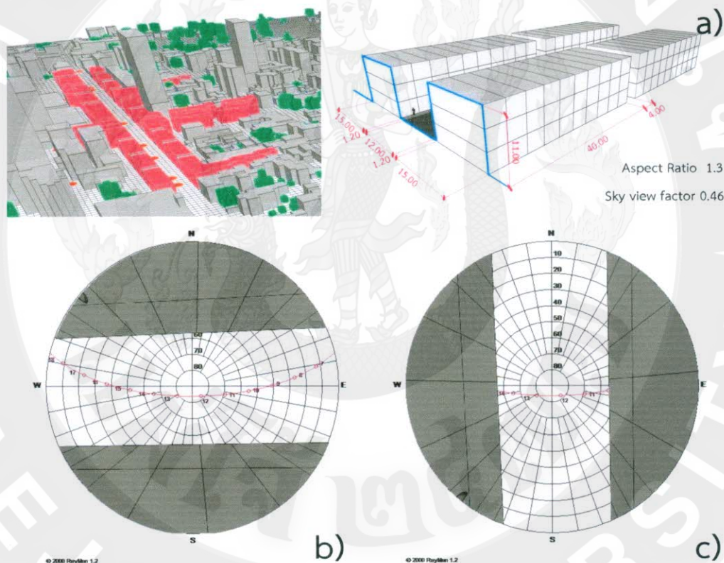
ภาพที่ 144 แสดงการปรับปรุงอาคารโดยอ้างอิงตามกฎหมายควบคุมอาคาร a) รูปทรงเรขาคณิตเมือง 1.3 b) Sky view factor บริเวณกลางถนนแนวทิศตะวันออก-ทิศตะวันตก C) Sky view factor บริเวณกลางถนนแนวทิศเหนือ-ทิศใต้ ที่มา : ผู้วิจัย
