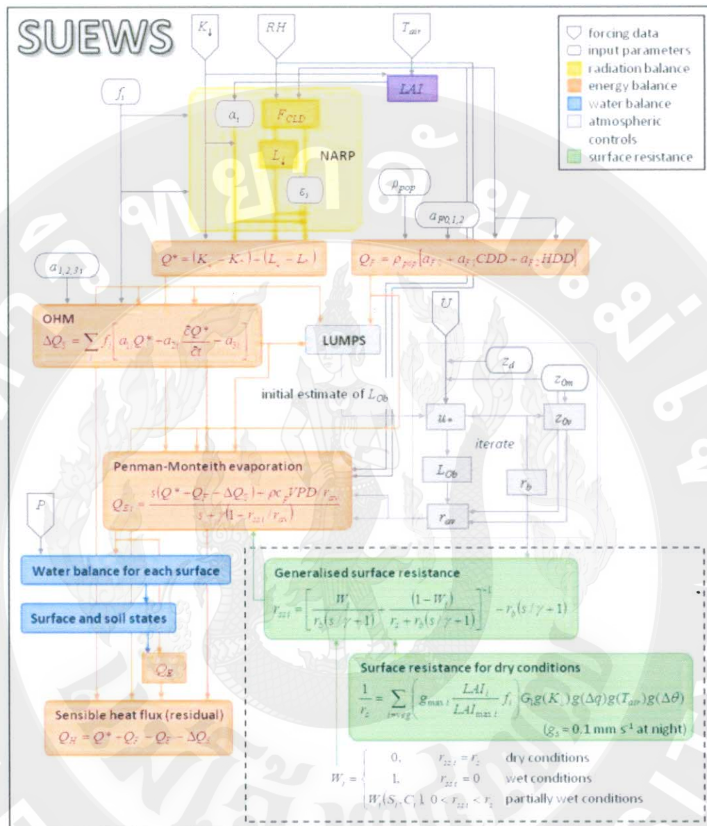
ภาพที่ 54 แผนผังแสดงโครงสร้างสมการแบบจำลอง SUEWS ภายในกริดเซลล์ ที่มา : Ward et al. (2016)
