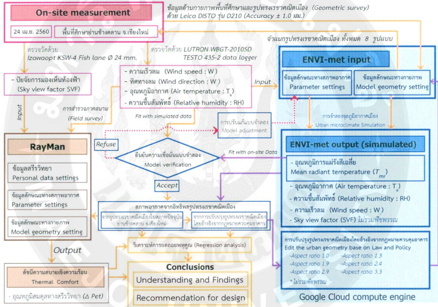
ภาพที่ 92 กระบวนการทางเทคนิคการวิจัย (Technical flow chart) ที่มา : ผู้วิจัย
