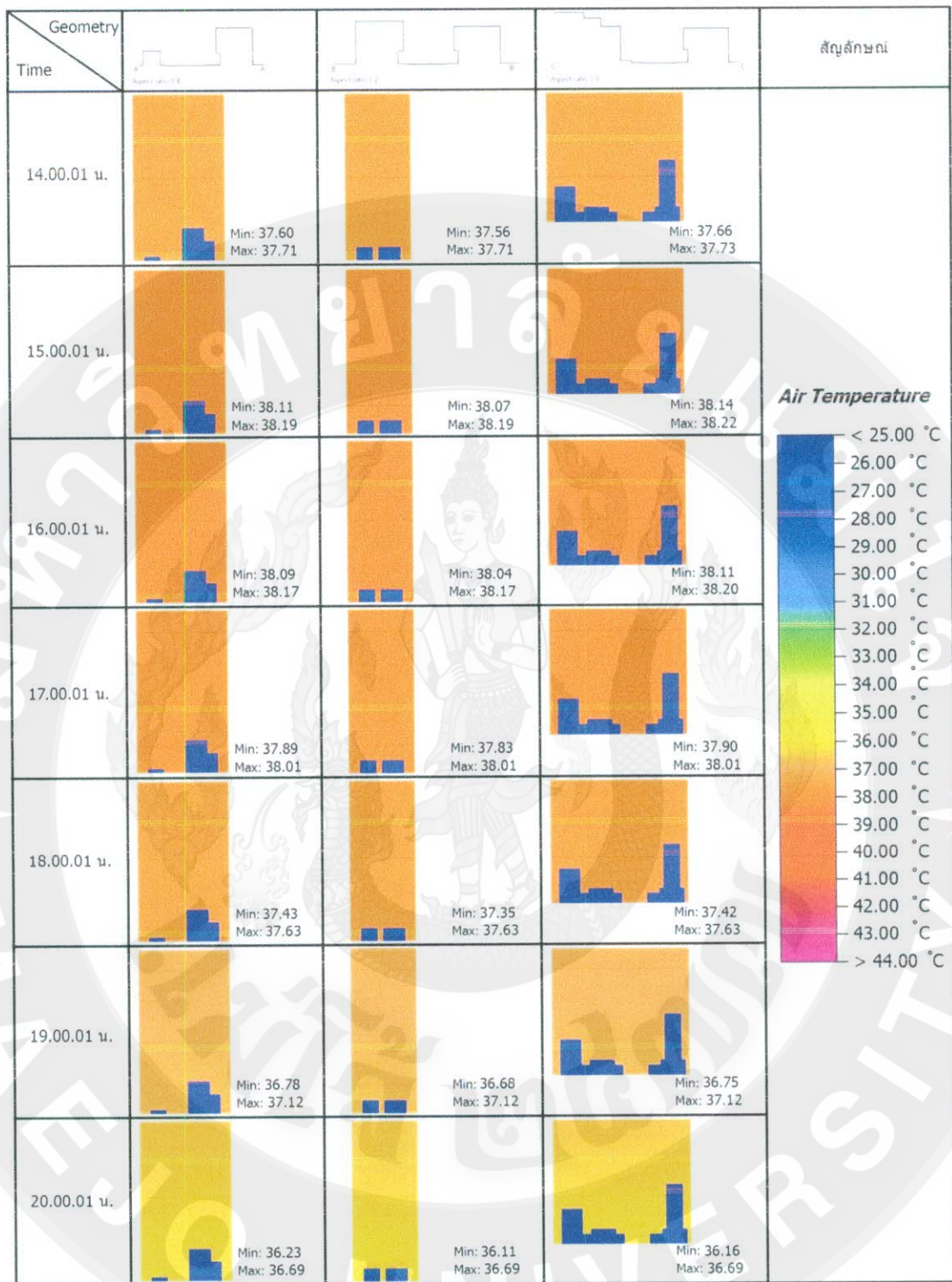
ภาพแสดงอุณหภูมิอากาศ(°C) ของรูปทรงเรขาคณิตเมือง0.8, 1.2 และ 1.0 ในสภาพปัจจุบัน บริเวณถนนเหนือพื้นดิน 1.80 เมตร ตามแนวนอนทิศเหนือ-ทิศใต้ เวลา 14.00-20.00 น.
