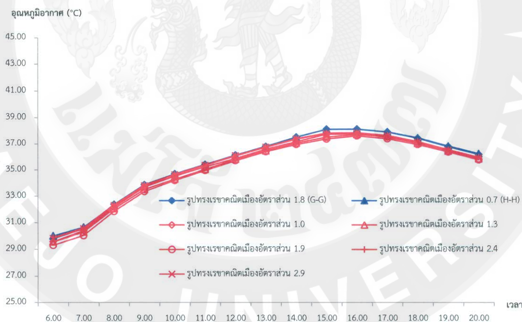
ภาพที่ 149 แสดงการเปรียบเทียบการเปลี่ยนแปลงอุณหภูมิอากาศ ในช่วงเวลา 6.00 – 20.00 น. ระหว่างรูปทรงเรขาคณิตเมืองในสภาพปัจจุบัน และปรับปรุงรูปทรงเรขาคณิตเมือง ในแนวนอนทิศตะวันออก – ทิศตะวันตก
