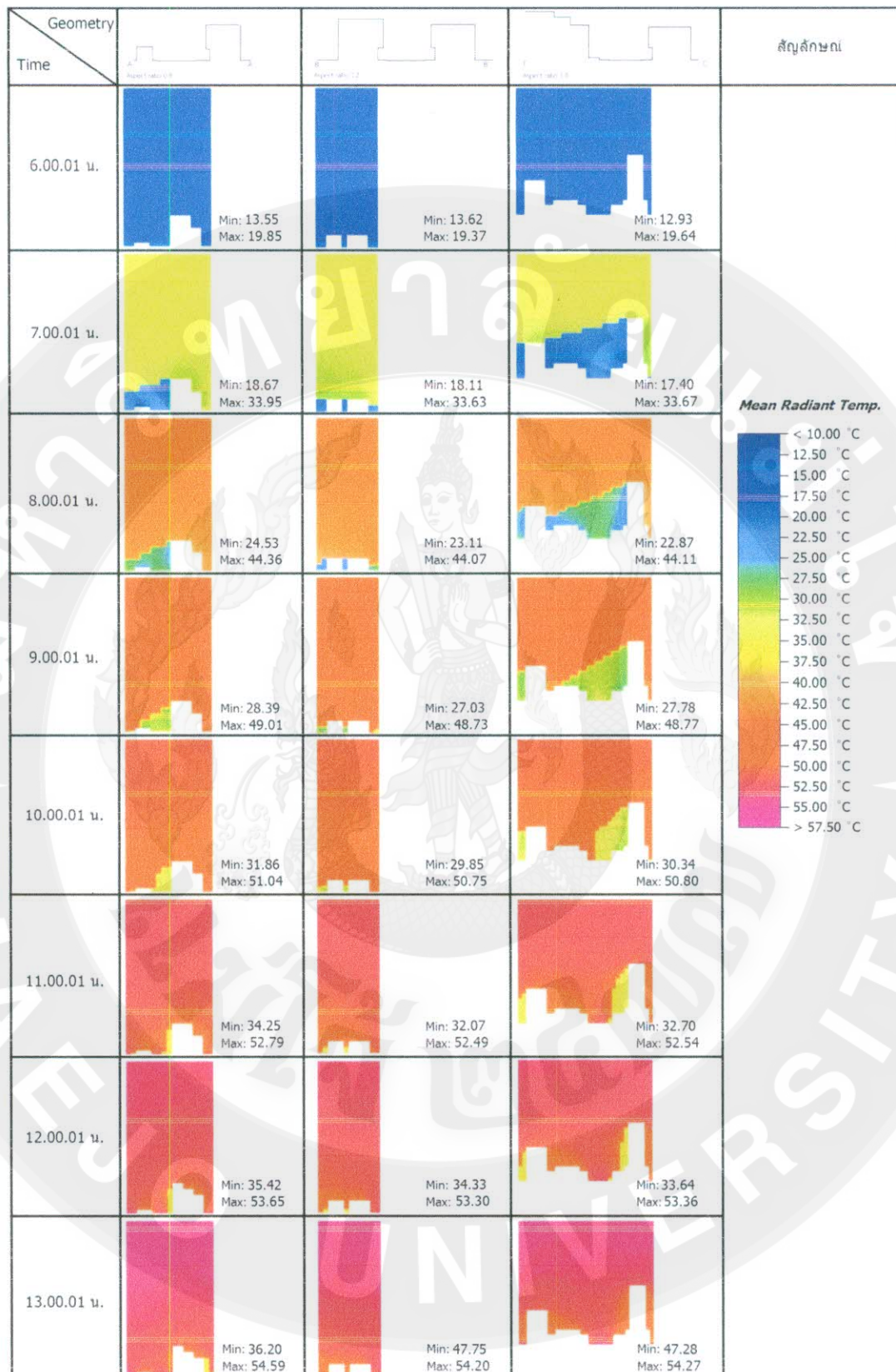
ภาพแสดงอุณหภูมิการแผ่รังสีเฉลี่ย(°C) ของรูปทรงเรขาคณิตเมือง 0.8, 1.2 และ 1.0 ในสภาพปัจจุบัน บริเวณถนนเหนือพื้นดิน 1.80 เมตร ตามแนวนอนทิศเหนือ-ทิศใต้ เวลา 6.00-13.00 น.
