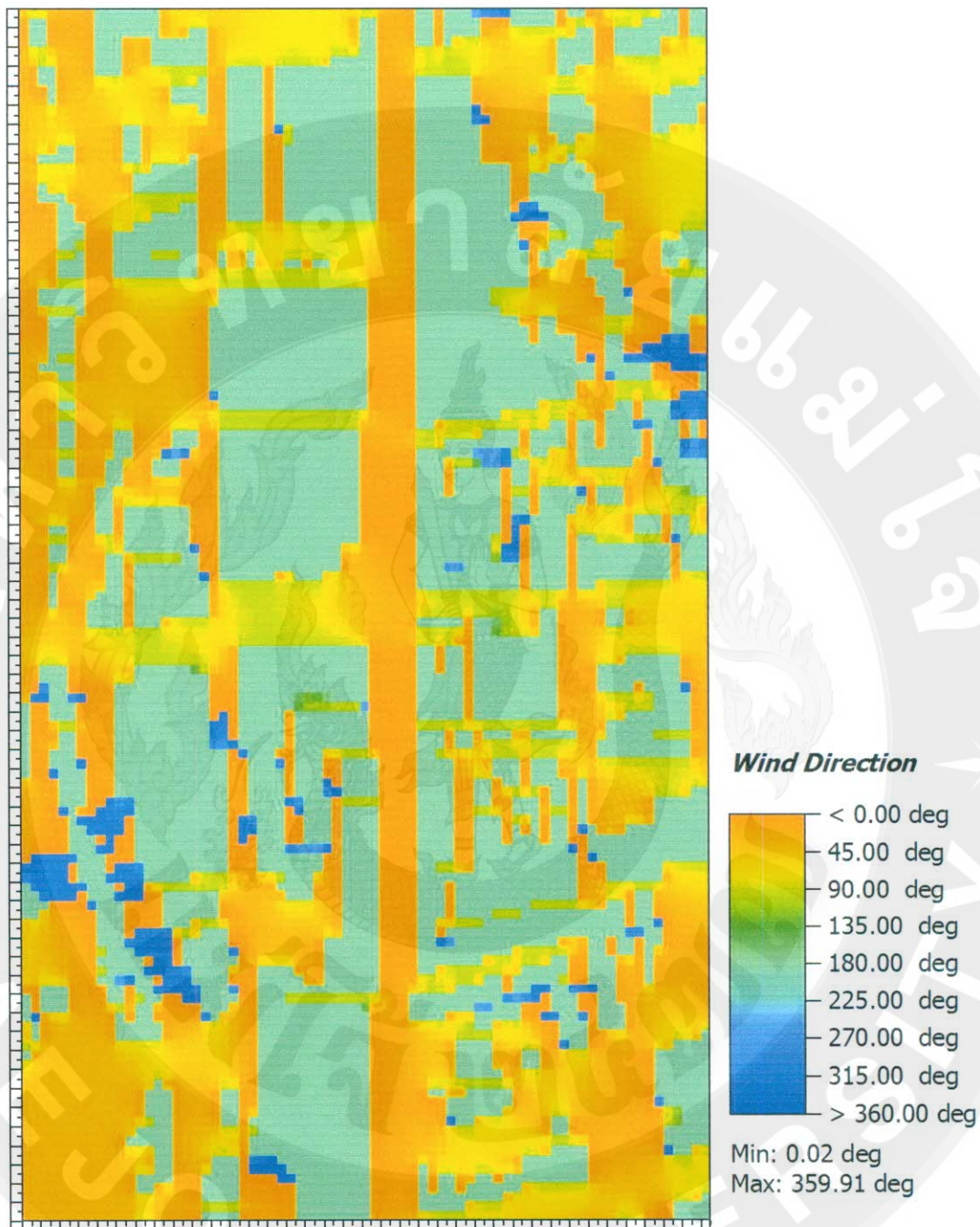
ภาพที่ 135 แสดงการจำลองทิศทางลมในพื้นที่ศึกษาย่านช้างคลาน ในวันที่ 24 เมษายน 256 เวลา 16.00 น.
