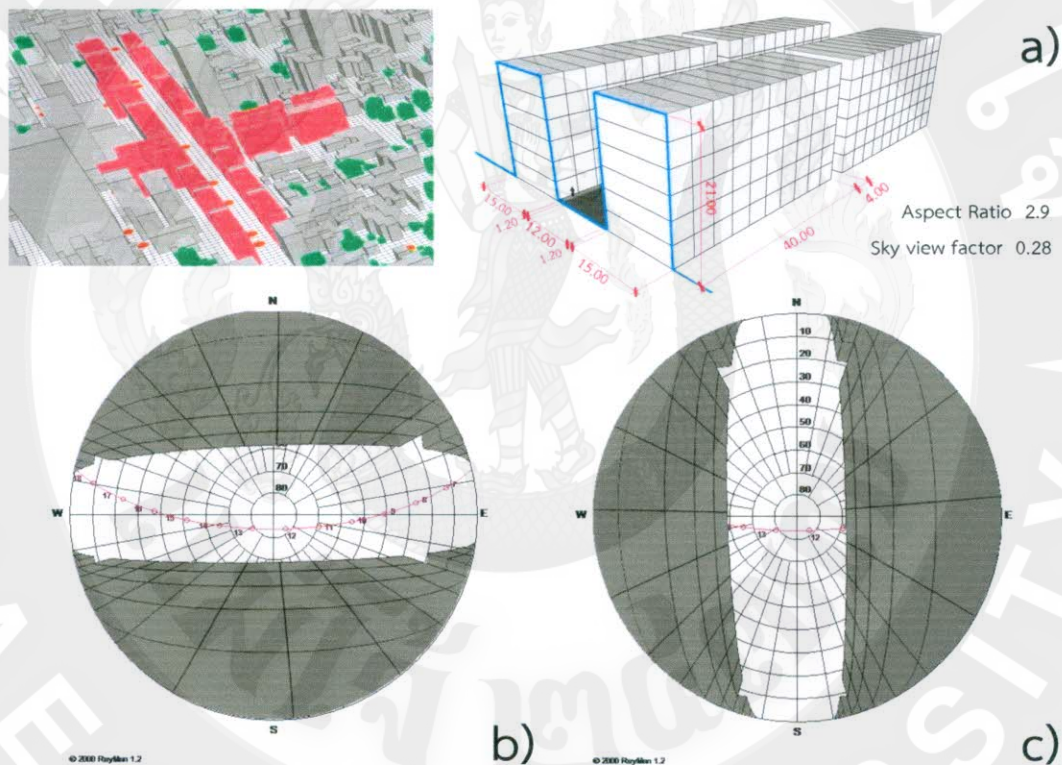
ภาพที่ 147 แสดงการปรับปรุงอาคารโดยอ้างอิงตามกฎหมายควบคุมอาคาร a) รูปทรงเรขาคณิตเมือง 2.9 b) Sky view factor บริเวณกลางถนนแนวทิศตะวันออก-ทิศตะวันตก c) Sky view factor บริเวณกลางถนนแนวทิศเหนือ-ทิศใต้
