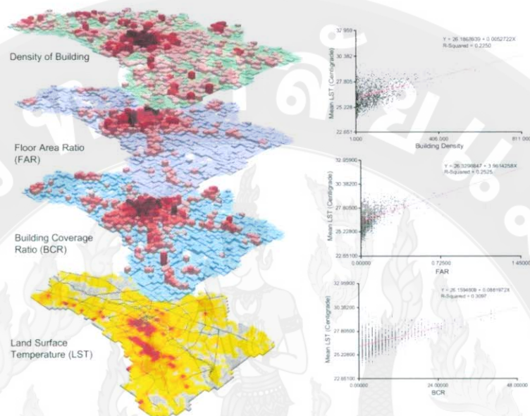
ภาพที่ 33 ภาพแสดงการวิเคราะห์ความสัมพันธ์ระหว่างอุณหภูมิพื้นผิวเมืองเชียงใหม่ กับความหนาแน่นอาคาร อัตราส่วนพื้นที่อาคารรวมต่อพื้นที่ดิน และอัตราส่วนพื้นที่อาคารปกคลุมดินต่อพื้นที่ดิน
