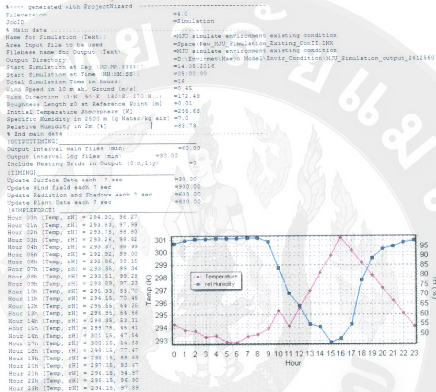
ภาพที่ 8 แสดงการตั้งค่าแบบจำลองสภาพภูมิอากาศภายในโปรแกรม Envi-met V.4
