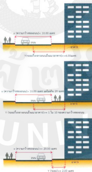
ภาพที่ 63 ระยะร่นของอาคารจากแนวถนนสาธารณะ ทั้ง 3 กรณี ที่มา : ผู้วิจัย
