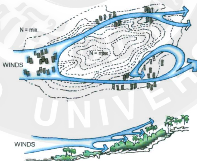
ภาพที่ 6 การระบายอากาศในลักษณะภูมิประเทศที่แตกต่างกัน ที่มา : Givoni (1998)
