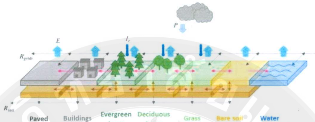
ภาพที่ 55 แสดงลักษณะพื้นผิวเมืองทั้ง 7 พื้นผิว ของแบบจำลอง SUEWS ที่มา : Järvi et al. (2011)
