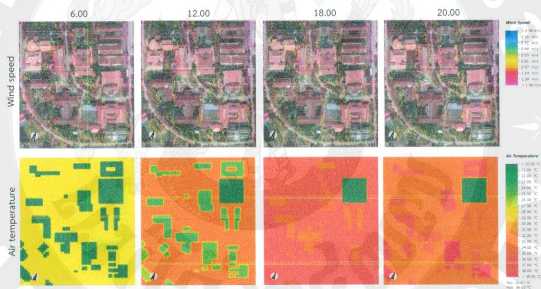
ภาพที่ 11 แสดงรูปแบบการไหลเวียนอากาศ ความเร็วลม (m/s) และอุณหภูมิอากาศ (°C) ในกรณีการเปิดช่องระบายอากาศบางส่วนในพื้นที่ชั้นหนึ่งของอาคาร
