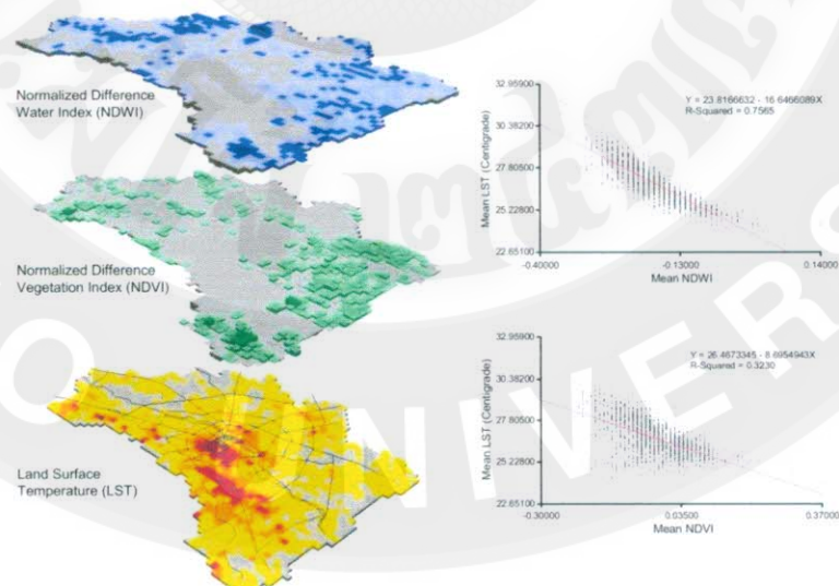
ภาพที่ 34 ภาพแสดงการวิเคราะห์ความสัมพันธ์ระหว่างอุณหภูมิพื้นผิวเมืองเชียงใหม่ กับดัชนีผลต่งน้ำ (NDWI), ดัชนีผลต่งพืชพรรณ(NDVI)
