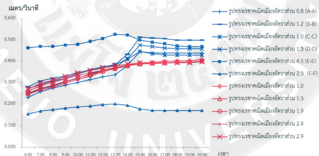
ภาพที่ 152 แสดงการเปรียบเทียบการเปลี่ยนแปลงความเร็วลม ในช่วงเวลา 6.00 – 20.00 น. ระหว่างรูปทรงเรขาคณิตเมืองในสภาพปัจจุบัน และปรับปรุงรูปทรงเรขาคณิตเมือง ในแนวนอนทิศ เหนือ – ทิศใต้
