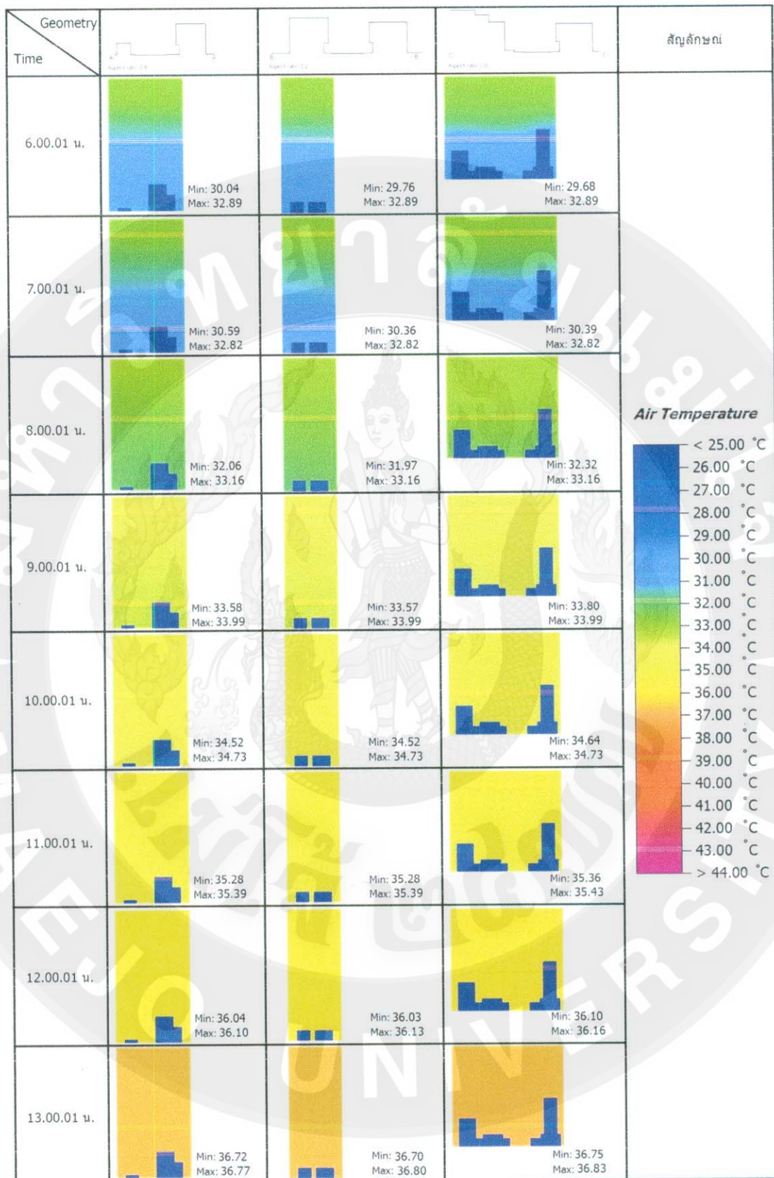
ภาพแสดงอุณหภูมิอากาศ(°C) ของรูปทรงเรขาคณิตเมือง 0.8, 1.2 และ 1.0 ในสภาพปัจจุบัน บริเวณถนนเหนือพื้นดิน 1.80 เมตร ตามแนวถนนทิศเหนือ-ทิศใต้ เวลา 6.00-13.00 น.
