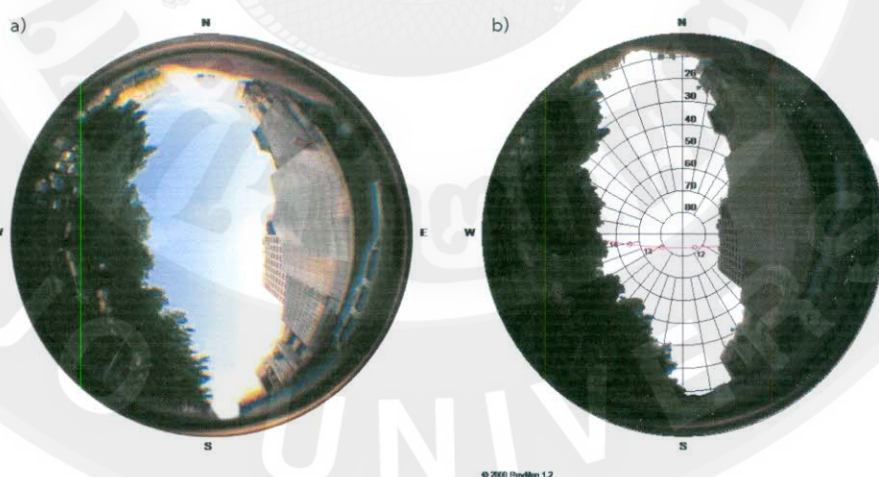
ภาพที่ 111 a) Sky view factor บริเวณกลางถนนของรูปทรงเรขาคณิตเมืองอัตราส่วน 0.30 b) ช่วงเวลาได้รับแสงอาทิตย์ของจุดรูปทรงเรขาคณิตเมืองอัตราส่วน 1.0 ที่มา : ผู้วิจัย
