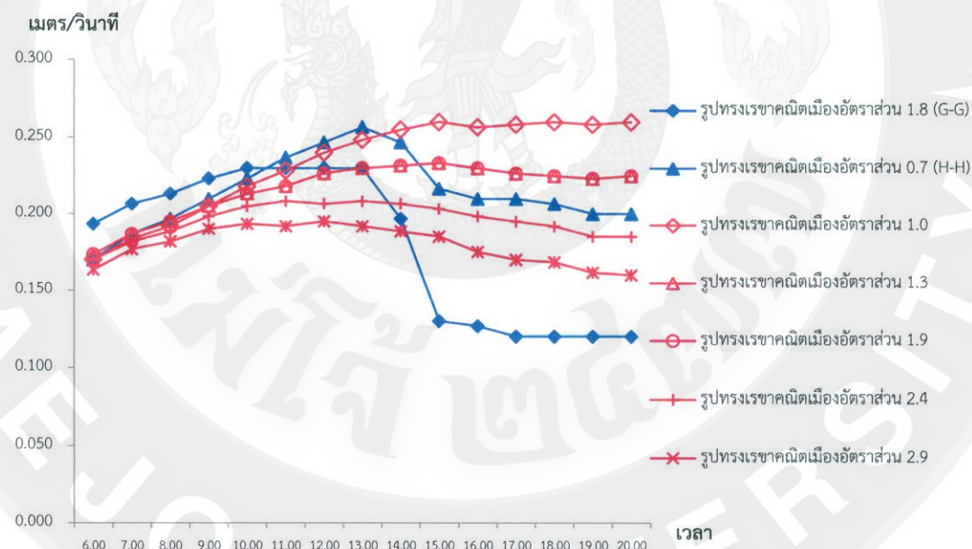
ภาพที่ 153 แสดงการเปรียบเทียบการเปลี่ยนแปลงความเร็วลม ในช่วงเวลา 6.00 – 20.00 น. ระหว่างรูปทรงเรขาคณิตเมืองในสภาพปัจจุบัน และปรับปรุงรูปทรงเรขาคณิตเมือง ในแนวนอนทิศตะวันออก – ทิศตะวันตก
