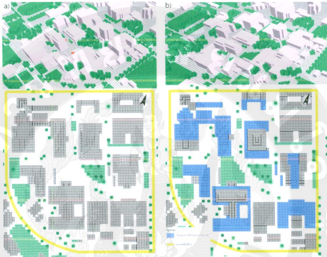
ภาพที่ 9 แสดงแบบจำลองทางกายภาพของพื้นที่เป็น 2 ลักษณะ a) ลักษณะอาคารในพื้นที่ตามสภาพปัจจุบัน และ b) แก้ไขเรขาคณิตเมืองด้วยการเปิดชั้นใต้ทุนอาคารบางส่วน (พื้นที่สีฟ้าแสดงถึงลักษณะอาคารที่มีการเปิดใต้ทุนสูง 3 เมตรและ 4 เมตร)
