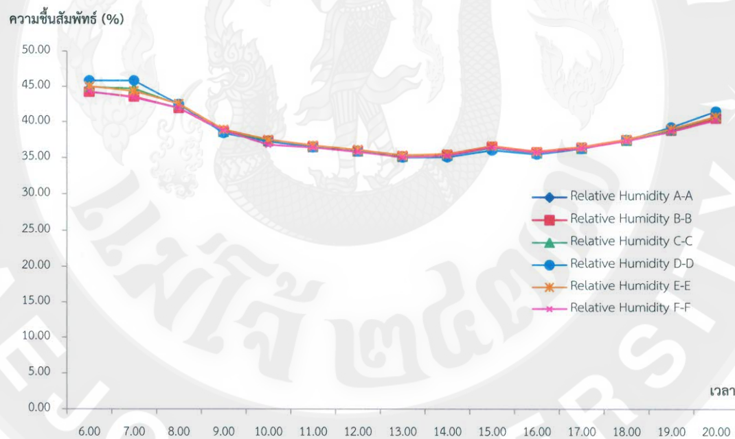
ภาพที่ 126 แสดงค่าความชื้นสัมพัทธ์ปัจจุบัน บริเวณจุดตัวอย่างรูปทรงเรขาคณิตเมือง ตามแนวถนนเหนือ - ใต้
