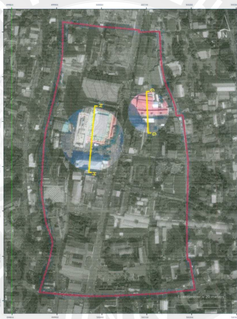
ภาพที่ 118 ภาพแสดงอัตราส่วนความสูงของอาคารต่อความกว้างถนนตามแนวถนนตะวันออก-ตะวันตก 2 รูปแบบ ที่มา : ผู้วิจัย
