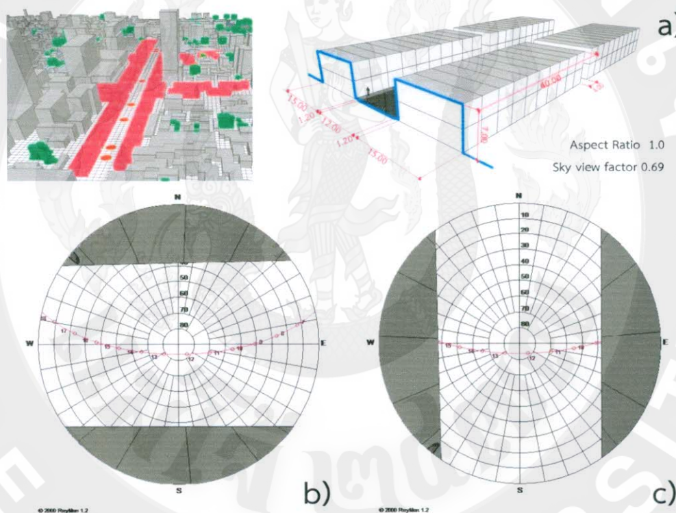
ภาพที่ 143 แสดงการปรับปรุงอาคารโดยอ้างอิงตามกฎหมายควบคุมอาคาร a) รูปทรงเรขาคณิตเมือง 1.0 b) Sky view factor บริเวณกลางถนนแนวทิศตะวันออก-ทิศตะวันตก c) Sky view factor บริเวณกลางถนนแนวทิศเหนือ-ทิศใต้
