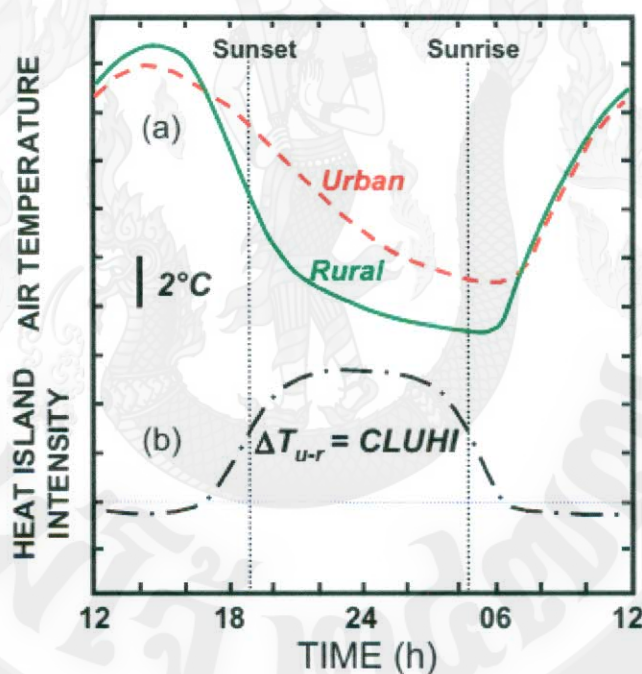
ภาพที่ 30 แผนภูมิแสดงการแปรเปลี่ยนของอุณหภูมิระหว่างวันในวันที่ท้องฟ้าปลอดโปร่ง ที่มา : Wong (2008)
