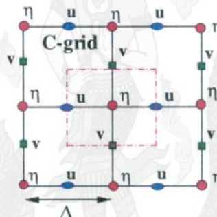
ภาพที่ 40 แสดงรูปแบบการคำนวณความต่างเชิงปริมาณของมุมฉากแบบ Arakawa C-grid ที่มา : Arakawa et al. (1977)
