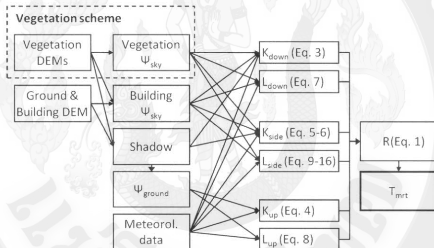
ภาพที่ 51 แสดงแผนผัง (Flowchart) การคำนวณของโปรแกรม SOLWEIG-model ซึ่ง \psi คือ ภาพของปัจจัยที่ใช้เป็นข้อมูลนำเข้าเพื่อใช้ในการคำนวณฟลักซ์ของรังสี ทั้ง 6 ทิศทาง ที่มา : Lindberg et al. (2011)
