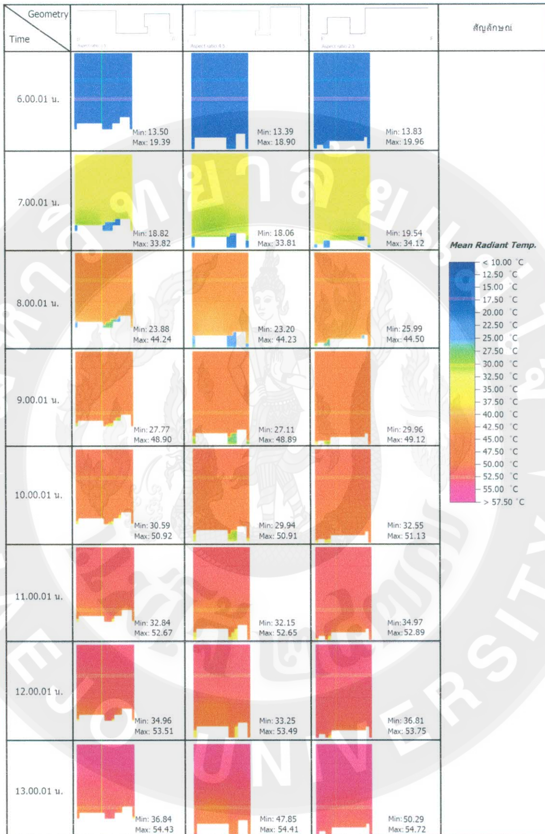
ภาพแสดงอุณหภูมิการแผ่รังสีเฉลี่ย(°C) ของรูปทรงเรขาคณิตเมือง 1.5, 4.5 และ 2.3 ในสภาพปัจจุบัน บริเวณถนนเหนือพื้นดิน 1.80 เมตร ตามแนวถนนทิศเหนือ-ทิศใต้ เวลา 6.00-13.00 น.
