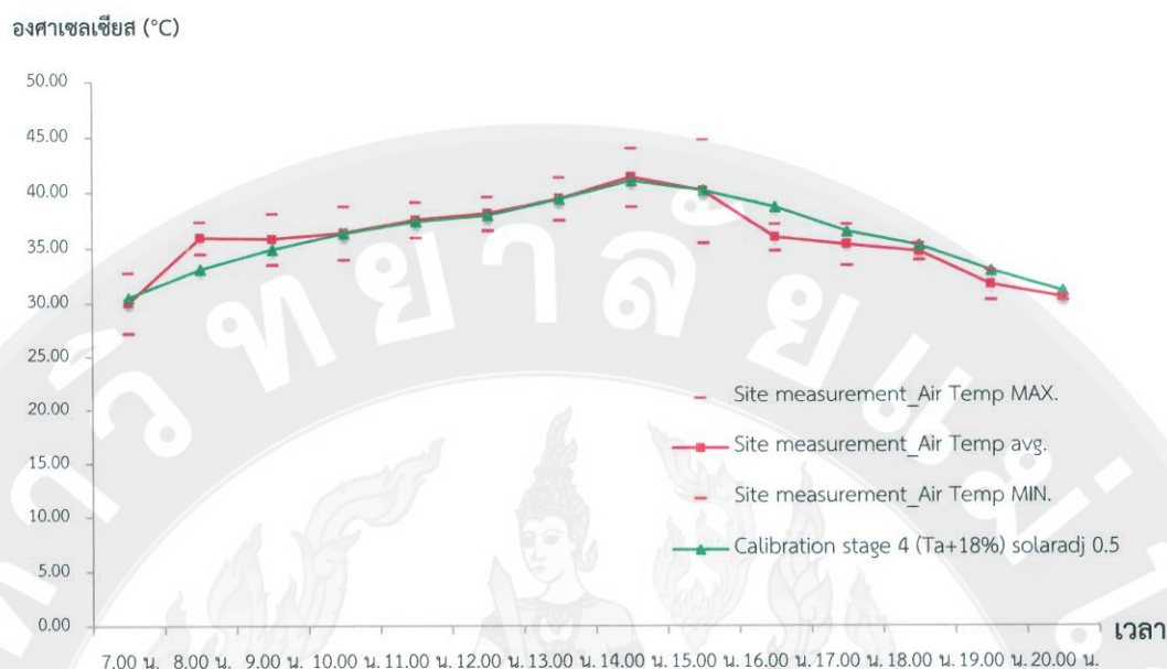
ภาพที่ 89 อุณหภูมิอากาศของแบบจำลองครั้งที่ 4 และอุณหภูมิอากาศของการตรวจวัดสภาพอากาศภาคสนาม ที่มา : ผู้วิจัย
