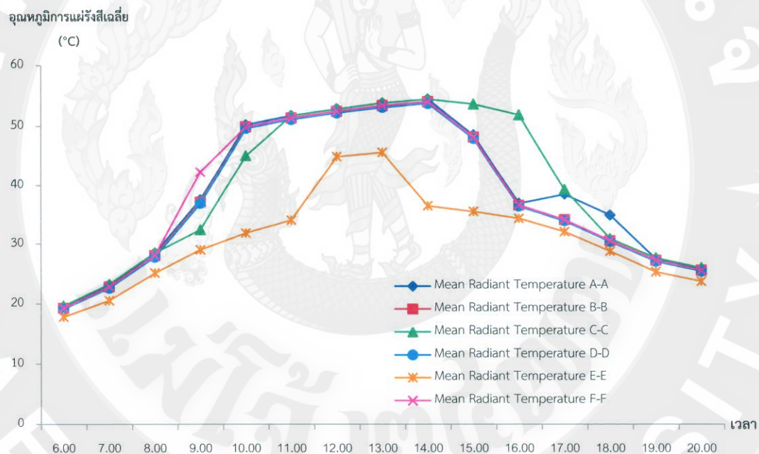
ภาพที่ 137 แสดงอุณหภูมิการแผ่รังสีเฉลี่ยปัจจุบัน บริเวณจุดตัวอย่างรูปทรงเรขาคณิตเมือง ตามแนวถนนเหนือ - ใต้
