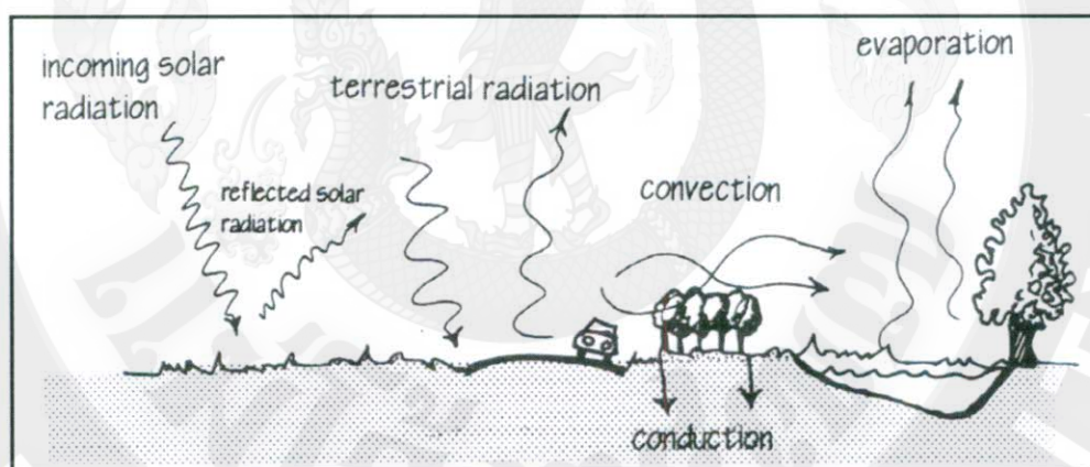
ภาพที่ 25 แสดงกระบวนการที่สำคัญที่มีอิทธิพลต่อการเปลี่ยนแปลงของอุณหภูมิอากาศเมือง
