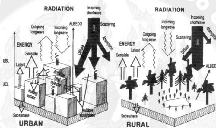
ภาพที่ 23 แสดงการเปรียบเทียบการแผ่รังสีจากแสงอาทิตย์ของพื้นที่เมืองและพื้นที่ชนบทในวันที่อากาศปลอดโปร่ง ที่มา : Oke (1987)
