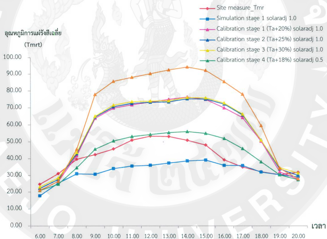
ภาพที่ 88 แสดงการเปรียบเทียบแนวโน้มค่าอุณหภูมิการแผ่รังสีเฉลี่ยของแบบจำลองกับการตรวจวัดภาคสนาม ณ จุดตรวจวัดสภาพอากาศ ที่มา : ผู้วิจัย
