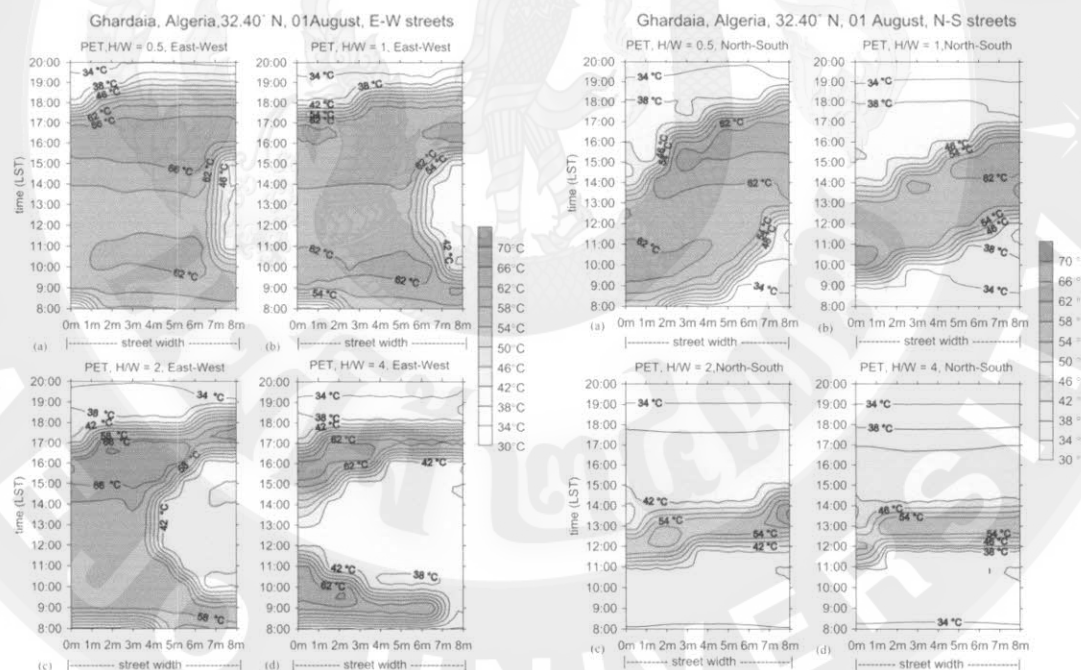
ภาพที่ 67 การเปลี่ยนแปลงเชิงพื้นที่และเวลาของอุณหภูมิเทียบเท่าทางสรีระวิทยา ตามทิศทางการวางตัวของอาคารแนวทิศเหนือ-ทิศใต้ และ ทิศตะวันออก - ทิศตะวันตก ของรูปทรงเรขาคณิตเมือง 0.5, 1, 2 และ 4
