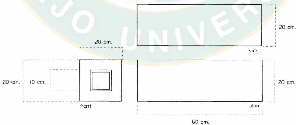
ภาพที่ 85 ภาพแปลนของวัตถุคอนกรีตมวลเบาแบบที่ 2.2
