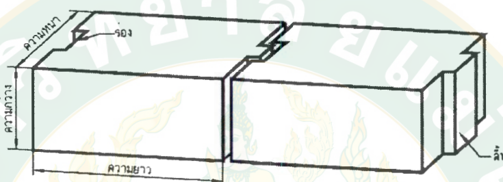
ภาพที่ 50 ภาพตัวอย่างข้อกำหนดลิ้นและร่องของคอนกรีตมวลเบา
