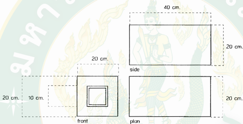
ภาพที่ 84 ภาพแปลนของวัตถุคอนกรีตมวลเบาแบบที่ 2.2
