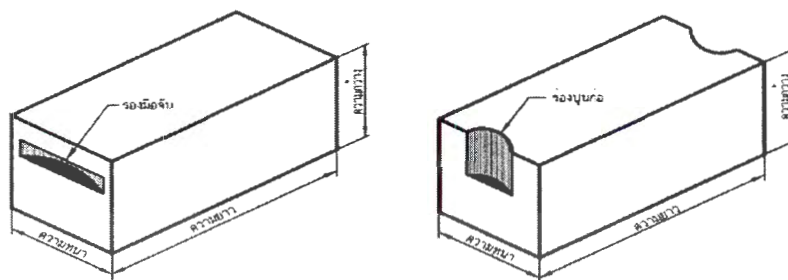
ภาพที่ 49 ภาพตัวอย่างข้อกำหนดร่องก่อและร่องมือจับ
