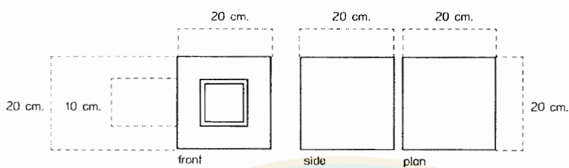
ภาพที่ 83 ภาพแปลนของวัตถุคอนกรีตมวลเบาแบบที่ 2.1
