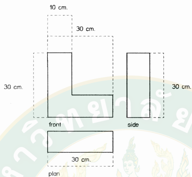
ภาพที่ 81 ภาพแปลนขนาดของวัสดุคอนกรีตมวลเบาแบบที่ 1.3
