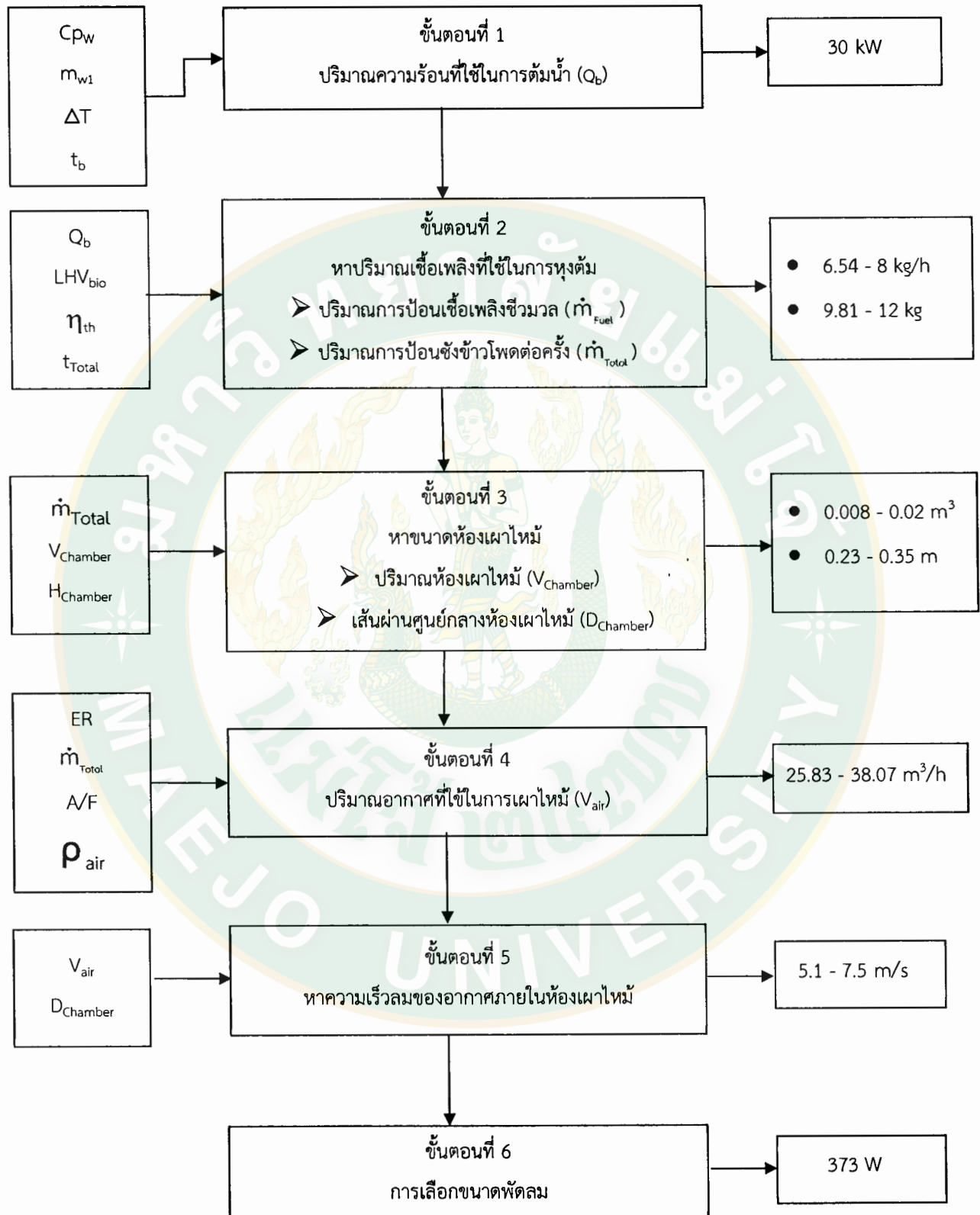
ภาพที่ 48 ไดอะแกรมการออกแบบเตาชีวมวล
