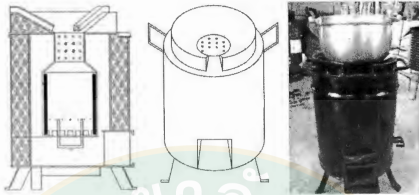
ภาพที่ 22 เตาแก๊สชีวมวลกรูทองเผาไหม้ประสิทธิภาพสูง
