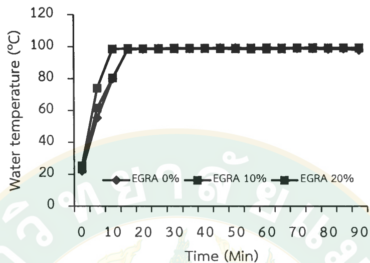
ภาพที่ 72 การปรับอัตราการป้อน EGRA ของซังข้าวโพดที่มีผลอุณหภูมิน้ำเดือด
