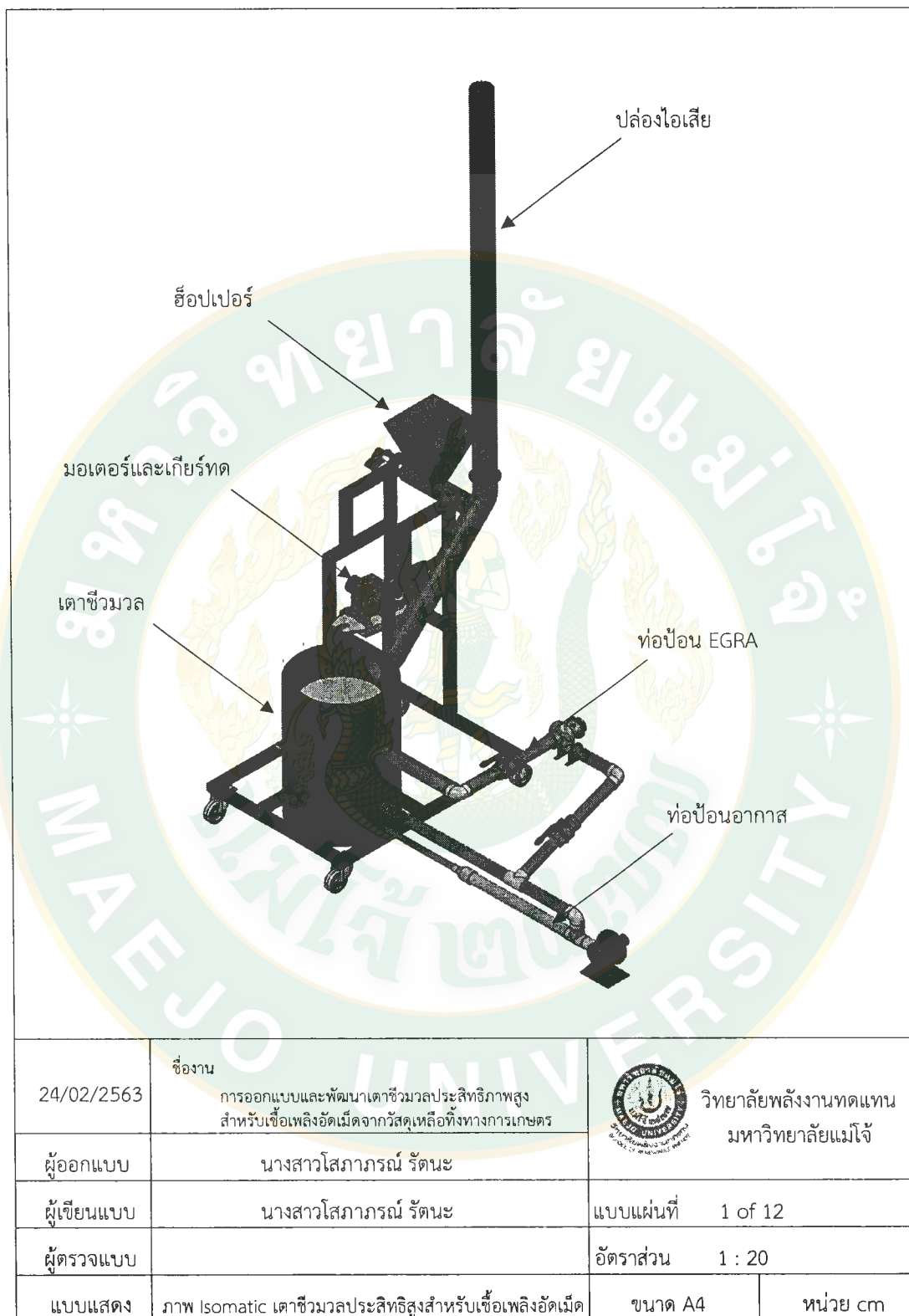
ภาพผนวกที่ 1 แบบเตาชีวมวลประสิทธิภาพสูง
