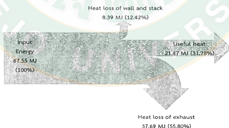
ภาพที่ 83 การสมดุลพลังงานของระบบเตาชีวมวลของการใช้เชื้อเพลิงฟางข้าว
