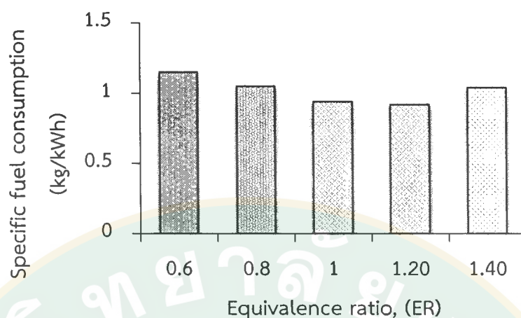
ภาพที่ 57 แสดงผลของอัตราส่วนสมมูลที่มีผลต่ออัตราการสิ้นเปลืองเชื้อเพลิงจำเพาะ
