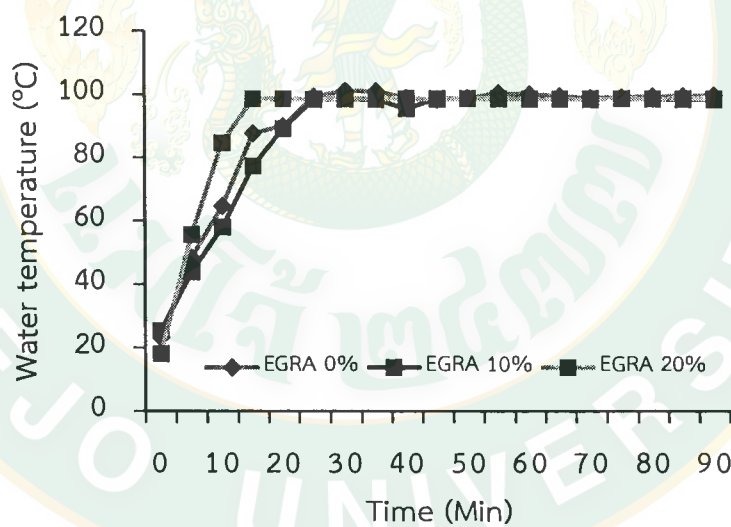
ภาพที่ 73 การปรับอัตราการป้อน EGRA ของเศษไม้ที่มีผลอุณหภูมิน้ำเดือด
