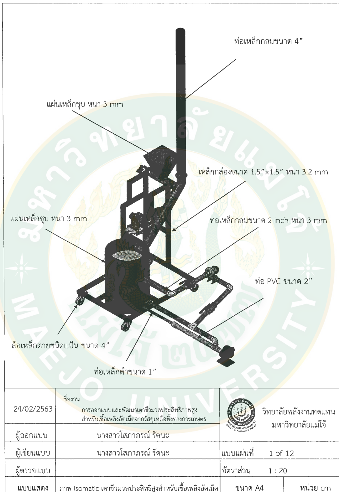
ภาพผนวกที่ 2 ส่วนประกอบเตาชีวมวลประสิทธิภาพสูง
