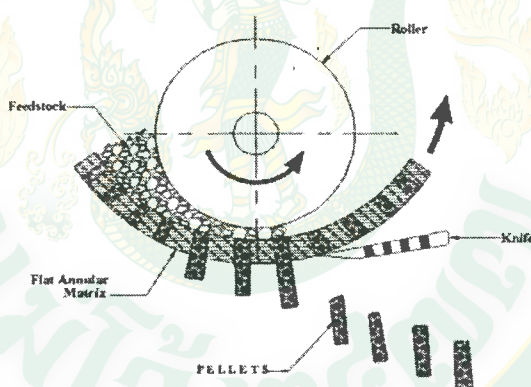
ภาพที่ 4 เครื่องอัดแบบแม่พิมพ์วงแหวน (Ring Palletizing press)
