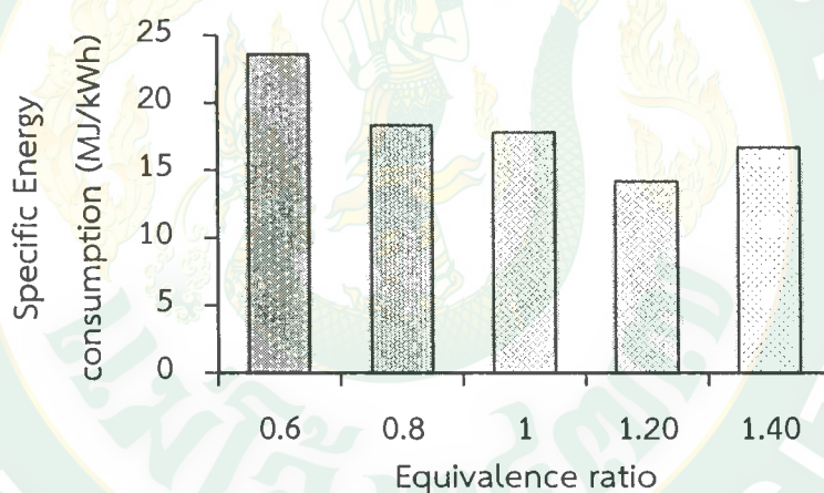
ภาพที่ 58 ผลของอัตราส่วนสมมูลที่มีผลต่ออัตราการสิ้นเปลืองพลังงานจำเพาะ
