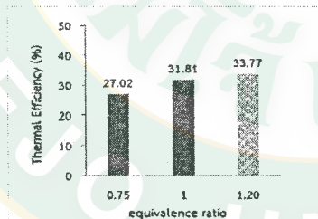
รูปที่ 6 ประสิทธิภาพความร้อนของเตาชีวมวลประสิทธิภาพสูง
