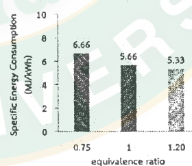
รูปที่ 4 อัตราการสิ้นเปลืองพลังงานจำเพาะ
