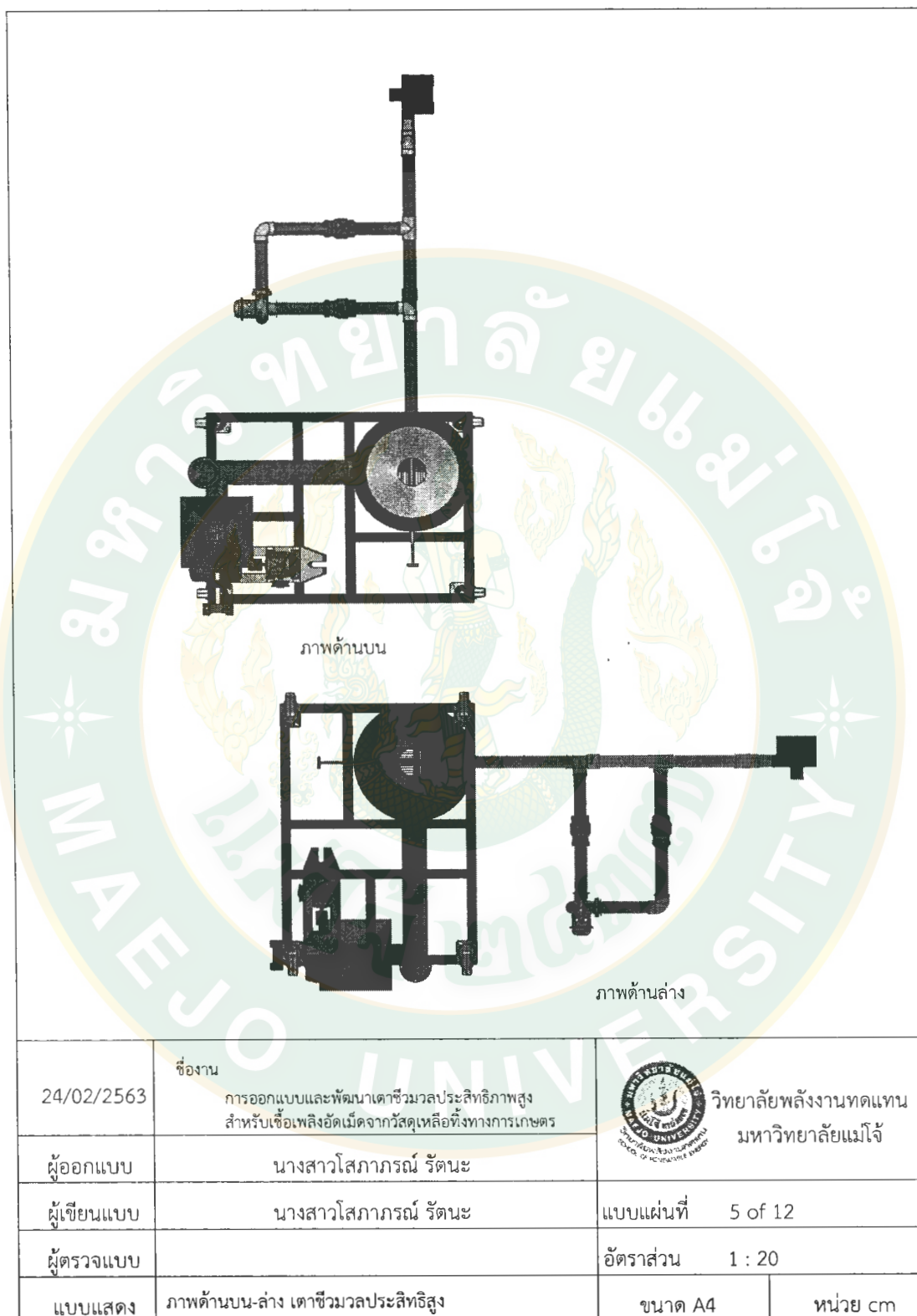
ภาพผนวกที่ 5 ภาพด้านบน-ล่าง เตาชีวมวลประสิทธิภาพสูง
