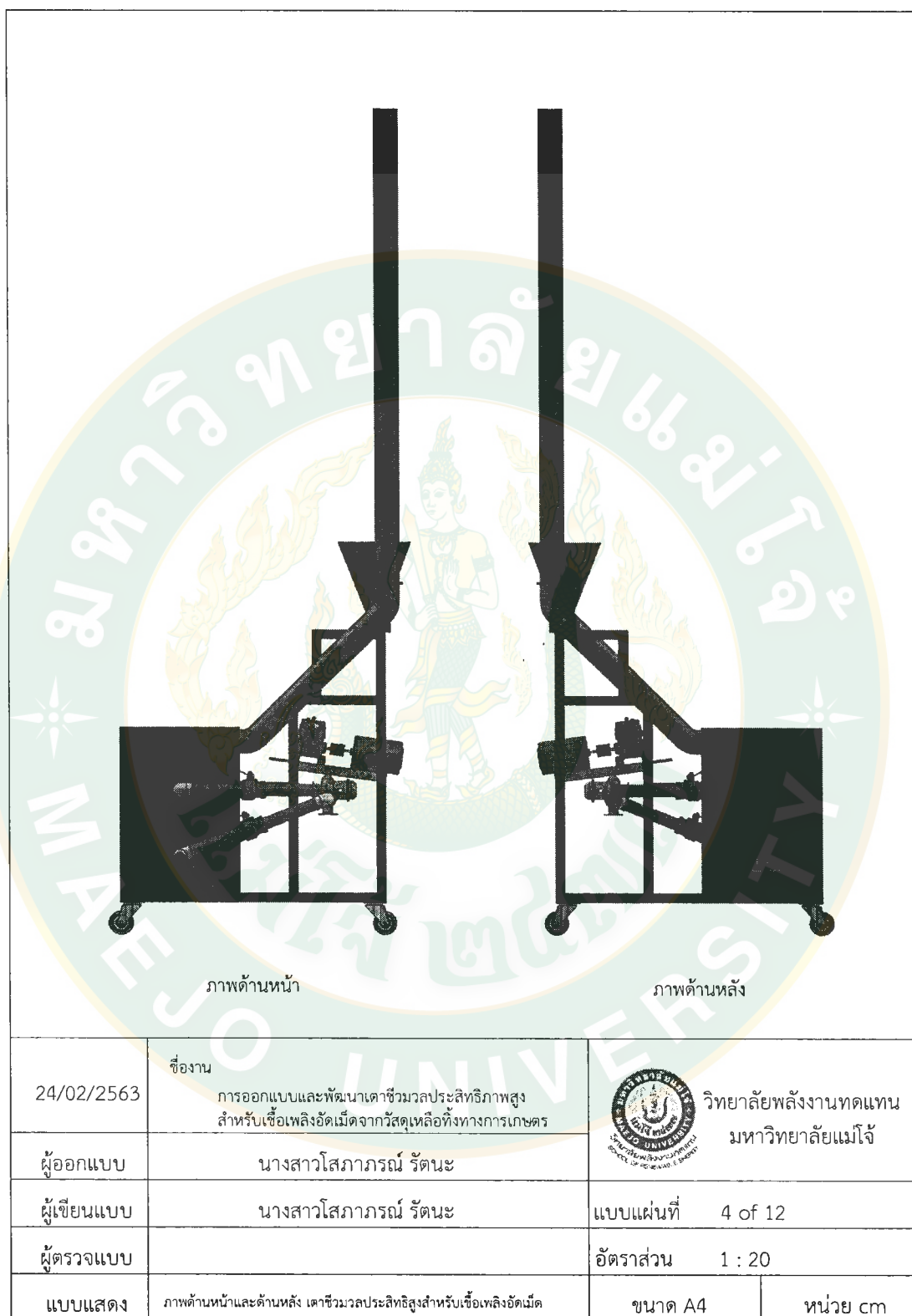
ภาพผนวกที่ 4 ภาพด้านหน้า-หลัง เตาชีวมวลประสิทธิภาพสูง
