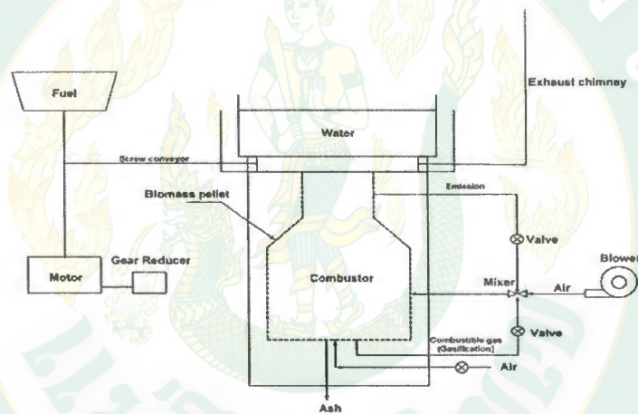
ภาพที่ 49 โครงสร้างเตาชีวมวลประสิทธิภาพสูง
