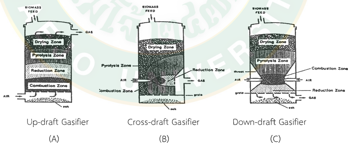
ภาพที่ 15 เครื่องผลิตโปรตีนเซอร์แก๊สแบบ Up-draft, Cross-draft และ Down-draft
