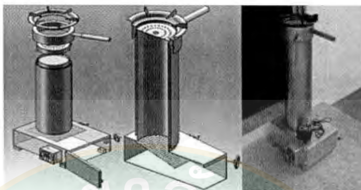
ภาพที่ 28 เตาแก๊สชีวมวลใช้วัสดุที่เหลือใช้ทางการเกษตรเป็นเชื้อเพลิง ที่มา: ณัฐวุฒิ ดุษฎี และคณะ (2551)
