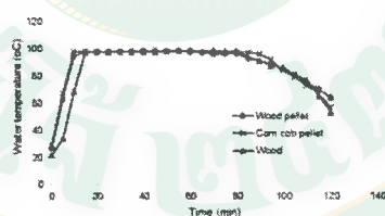
ภาพที่ 5 คุณสมบัติการเดือดของน้ำจากเตาชีวมวล
