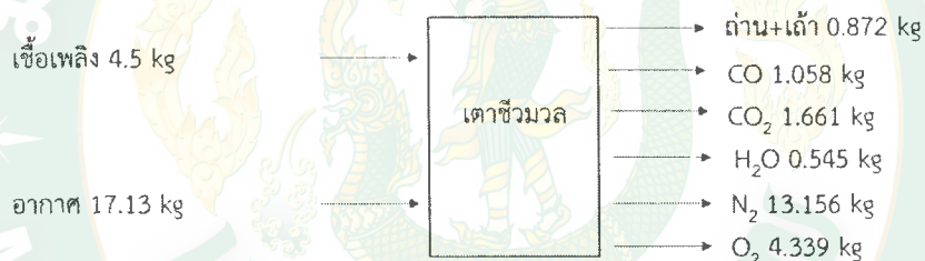
ภาพที่ 78 การสมดุลมวลของระบบเตาชีวมวลของการใช้เชื้อเพลิงซังข้าวโพด
