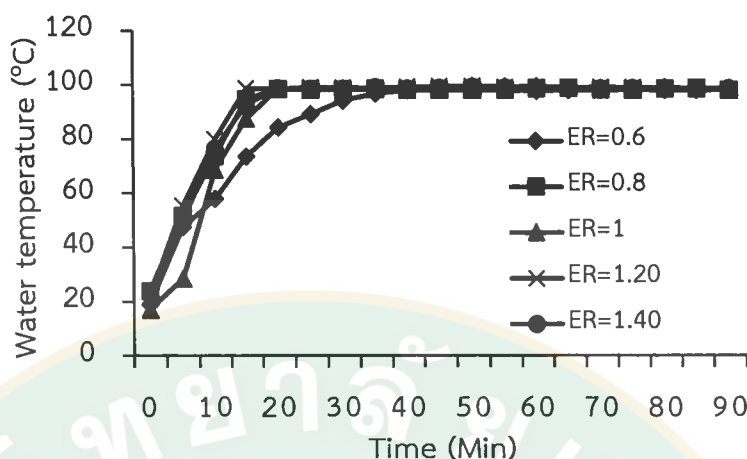
ภาพที่ 60 ผลของอัตราส่วนสมมูลที่มีผลต่ออุณหภูมิน้ำเดือด
