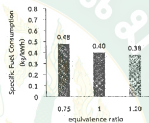
รูปที่ 3 อัตราการสิ้นเปลืองเชื้อเพลิงจำเพาะ
