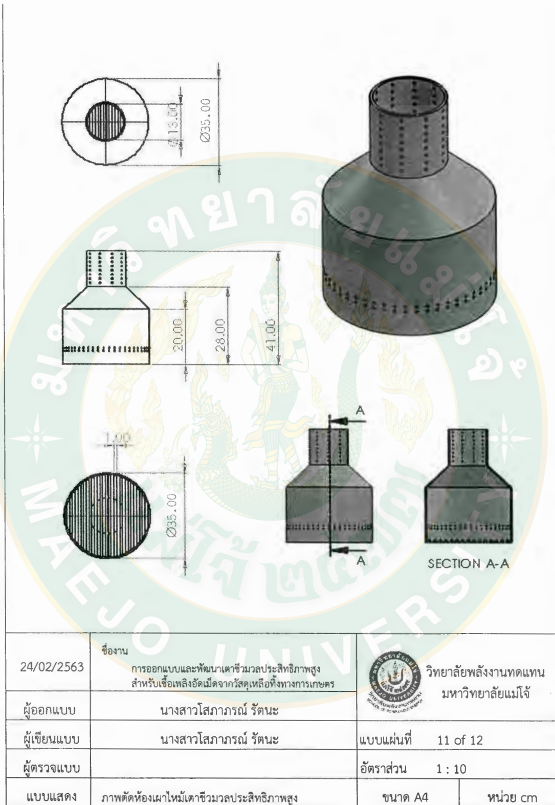
ภาพผนวกที่ 11 ชุดป้อนอากาศเตาชีวมวลประสิทธิภาพสูง
