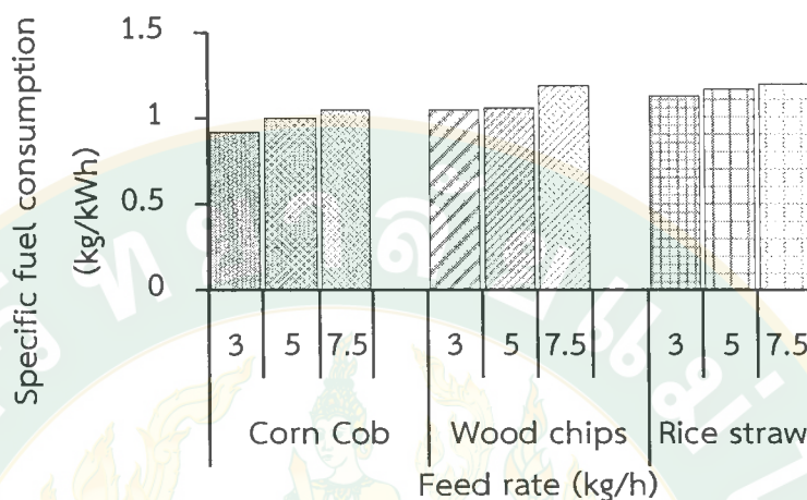
ภาพที่ 61 การปรับอัตราการป้อนเชื้อเพลิง ที่มีผลต่ออัตราการสิ้นเปลืองเชื้อเพลิงจำเพาะ
