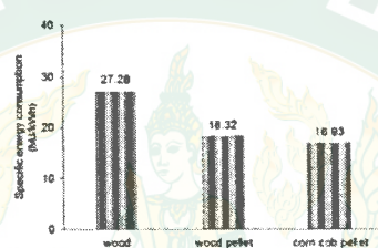
ภาพที่ 4 อัตราการใช้พลังงานจำเพาะ
