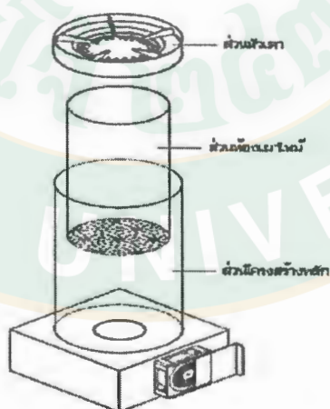
ภาพที่ 19 เตาหุงต้มเชื้อเพลิงแก๊ส
