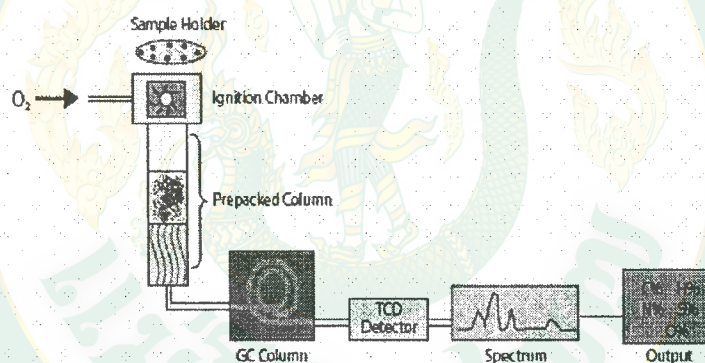
ภาพที่ 8 เครื่องวิเคราะห์ปริมาณธาตุ
