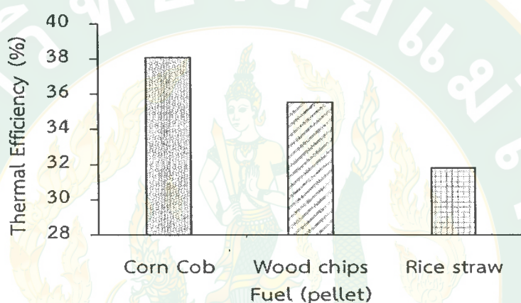
ภาพที่ 67 ผลของชนิดเชื้อเพลิงที่มีผลต่อประสิทธิภาพความร้อน
