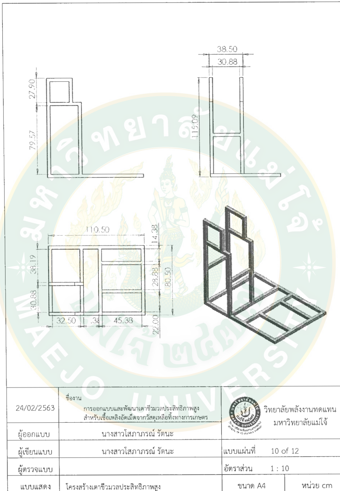
ภาพผนวกที่ 10 ชุดป้อนอากาศเตาชีวมวลประสิทธิภาพสูง
