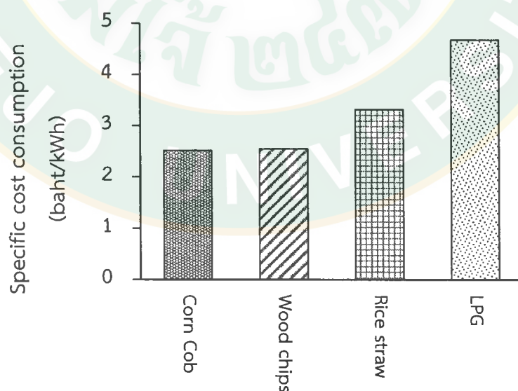
ภาพที่ 84 การประเมินต้นทุนการผลิตพลังงานความร้อน
